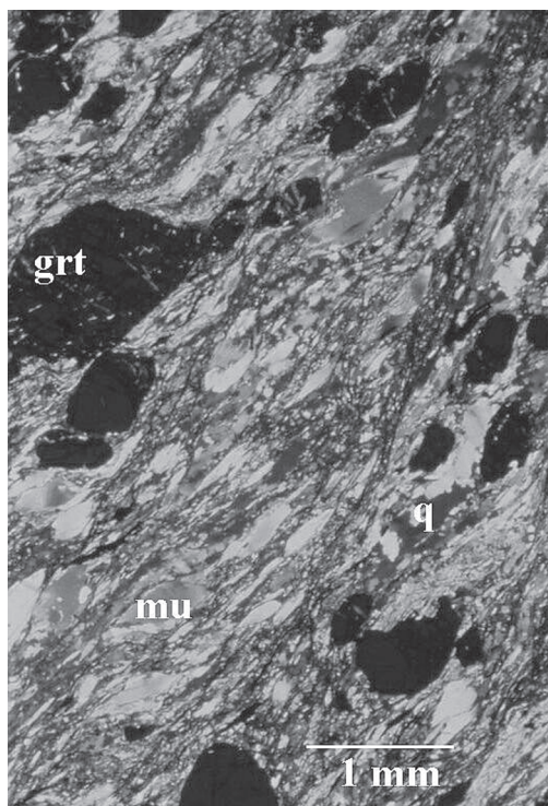
Sl. 5. Blastomilonitna struktura gnajsa z muskovitnimi ribicami. Vrtina MB-6, gl. 930 m, Muskovit (mu), granati (grt), kremen (q). MB-6, glob. 930 m.
