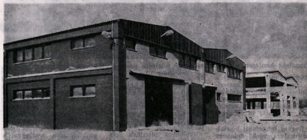
Proizvodne hale Juteks v Žalcu — grajene po montanžem sistemu Ingrad
