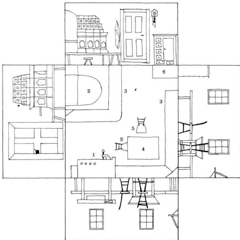
Slika 2. Notranja oprema »hiše« v Kartelovi kajži pred drugo vojno: 1. »verštat« – delovna miza, 2. peč, 3. klopi, 4. mentrga, 5. stola, 6. predalnik.
