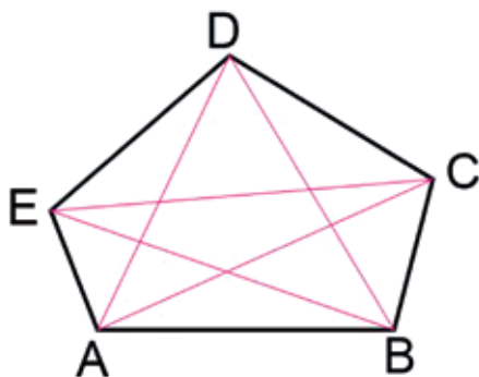
Slika 2: Konveksni petkotnik.
