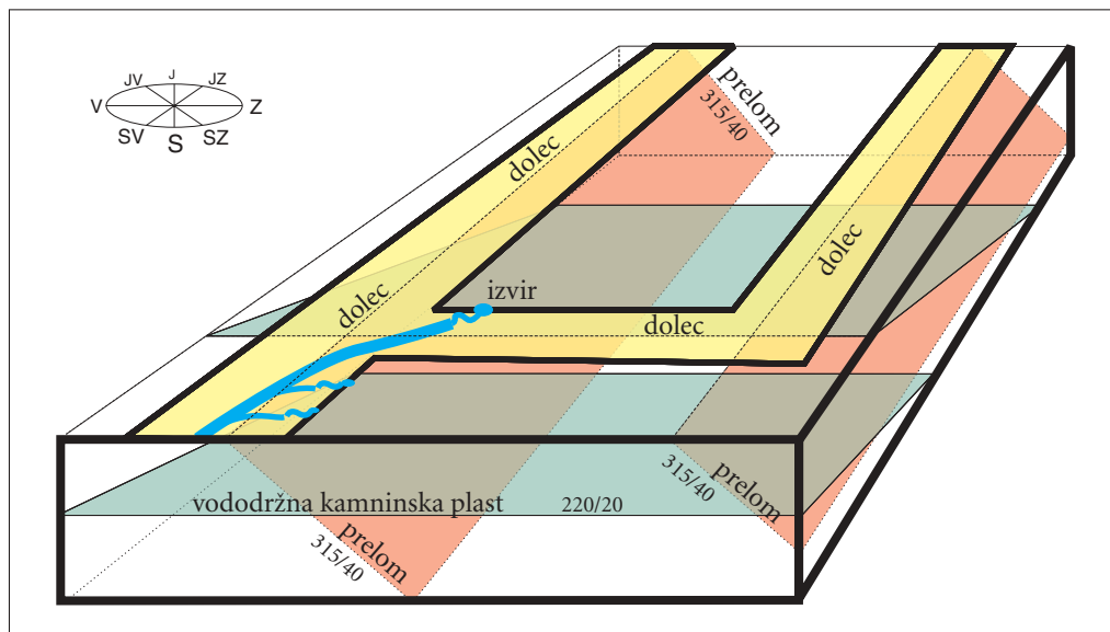
Slika 8: Geološko-strukturna podoba območja z dolci in lega izvira v Dolinah v Žibršah.
