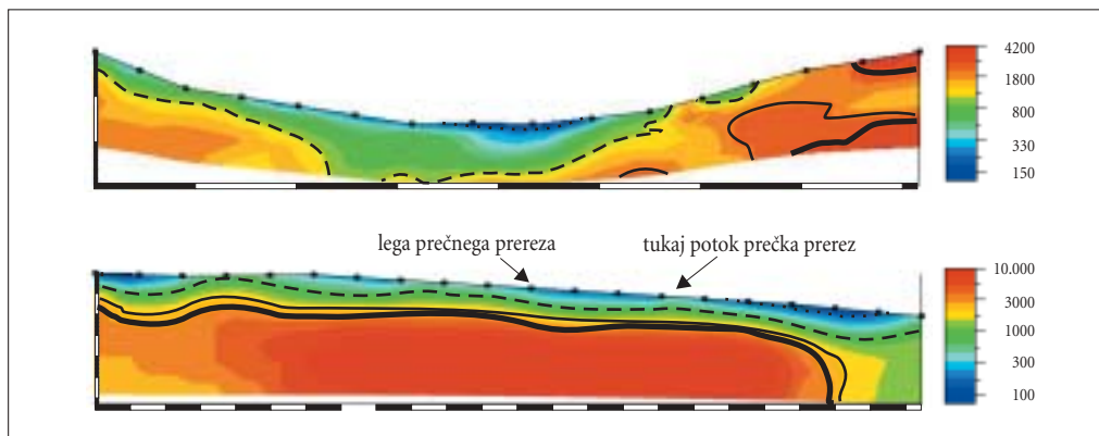
Slika 7: Vzdolžni prerez dolca, ki poteka vzdolž manj odpornih lapornatih plasti (spodaj) in prečni prerez čez isti dolec (zgoraj). Pikasta črna črta označuje predpostavljeno mejo med rdeče-rjavo ilovico in preperelo kamnino, ki je sredi dolca približno 2,5 m globoko. Debelino ilovice sem ugotovil z vrtnanjem. Črtkasta črta označuje predpostavljeno mejo med preperelo kamnino in močno razpokano kamnino. Polna črta označuje predpostavljeno mejo med razpokano in močno razpokano kamnino, debela polna črta pa predpostavljeno mejo med razpokano in nerazpokano kamnino, ugotovljeno z merjenjem elektroprevodnosti trdne kamnine. Z rdečo je obarvan kamninski blok v zaledju izvira. Navpični in vodoravni merila merita 5 m, elektroprevodnost je v \Omega m .
