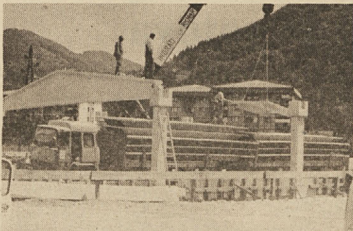
Detajl pri montaži stropnih PI plošč.
