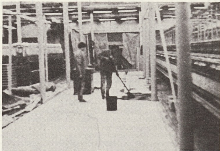
Polaganje parketa na temelje za 17. in 18. prstančni predilni stroj Textima.
