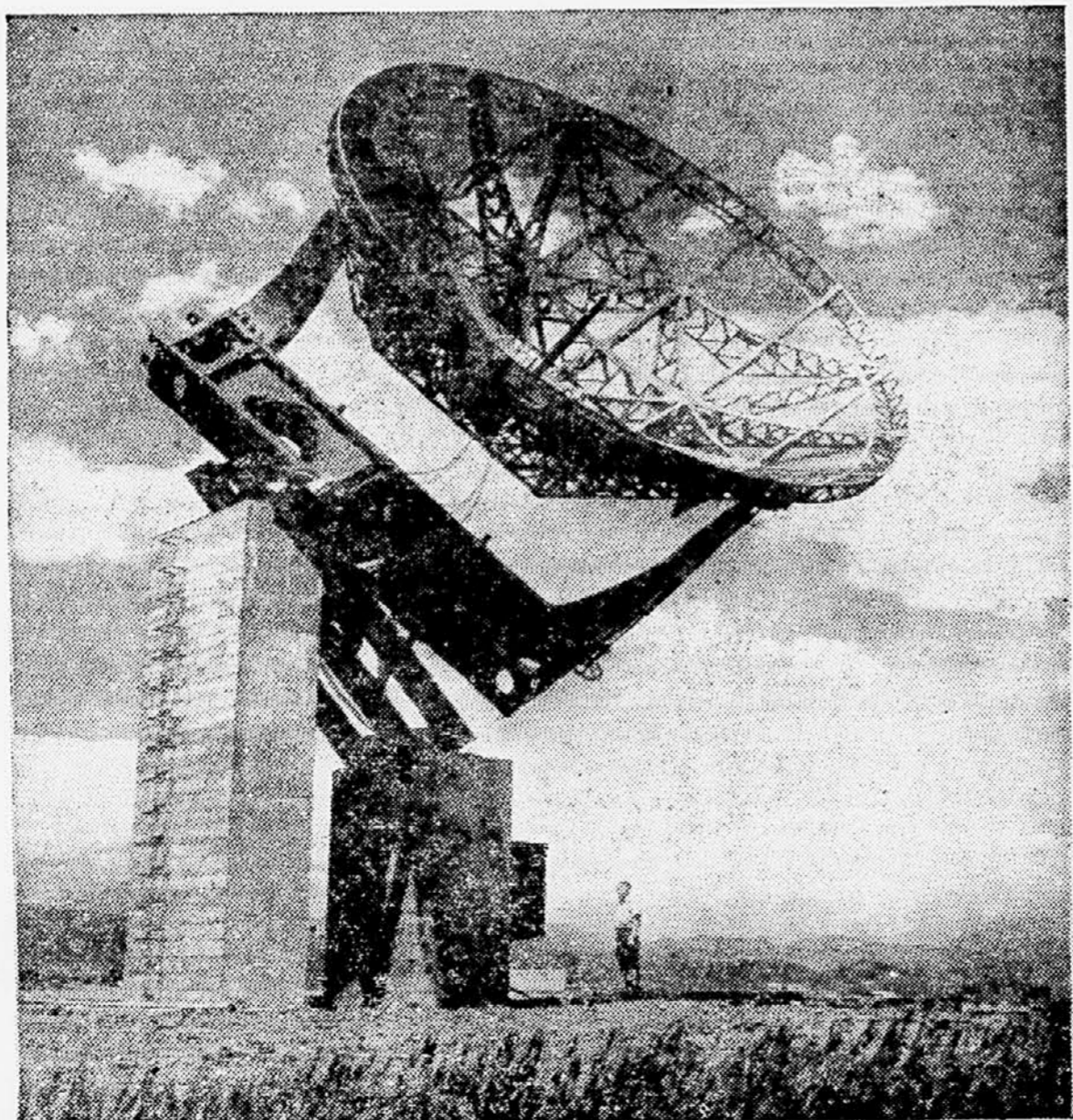
Ta ogromna »skodelca«, ki ima v premeru 7,6 m nima nobene zveze s prisluškovalno puško. To je radijski teleskop, s katerim znanstveniki v ZDA spremljajo sonce ter sprejemajo njegovo radijsko energijo in šume. V geofizičnem letu bo vrsta takih ogromnih teleskopov vsakodnevno merilo energije, ki jo oddaja sonce in registrirala sončne pege in druge motnje na soncu. Računajo, da bodo s pomočjo teh opazovanj dobili pomembne podatke o vplivu sonca na našo zemljo in na vreme.
