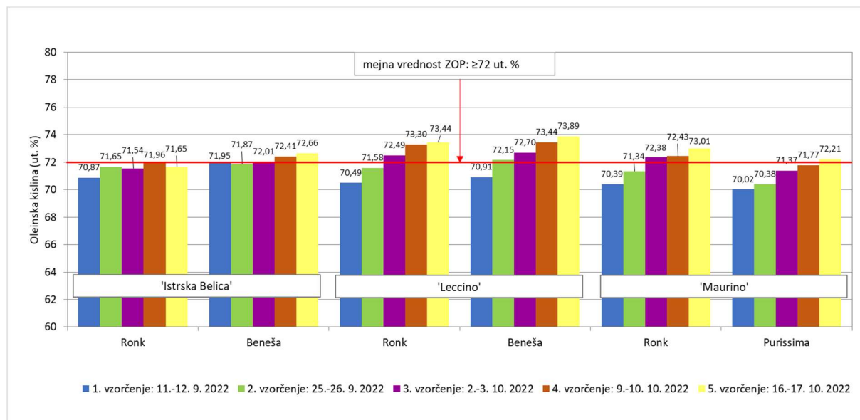
Slika 46: Vsebnost oleinske kisline v oljnih oljih sort 'Istrska Belica' in 'Leccino' na lokacijah Ronk in Beneša ter sorte 'Maurino' na lokacijah Ronk in Purissima; oljke so bile obrane v petih terminih vzorčenja
