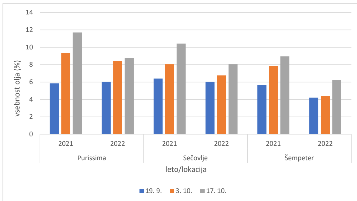
Slika 2: Vsebnost olja (%) sorte 'Mata' v laboratorijski oljarni (Abencor) v treh obdobjih vzorčenja v letih 2021 in 2022
