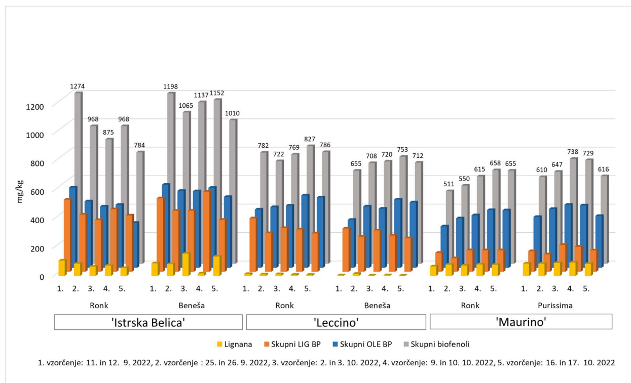
Slika 49: Primerjava vsebnosti lignanov, biofenolov ligostroziidnega (skupni LIG BP) in olevropeinskega izvora (skupni OLE BP) in skupnih biofenolov v oljčnih oljih iz sort 'Istrska Belica' in 'Leccino' na lokacijah Ronk in Beneša ter sorte 'Maurino' na lokacijah Ronk in Purissima; oljke so bile obrane v petih terminih vzorčenja.
