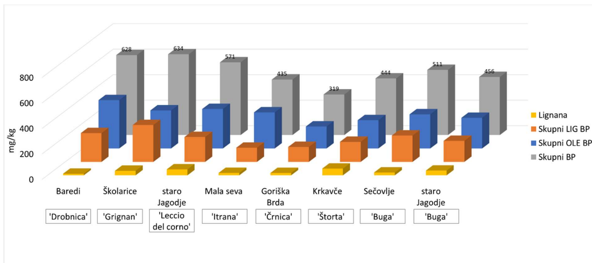
Slika 61: Primerjava vsebnosti lignanov, biofenolov ligostrozidnega (skupni LIG BP) in olevropeinskega izvora (skupni OLE BP) in skupnih biofenolov v oljčnih oljih sort 'Drobnica', 'Grignan', 'Leccio del corno', 'Itrana', 'Črnica', 'Štorta' in 'Buga' z različnih lokacij, predelanih v oktobru 2022
