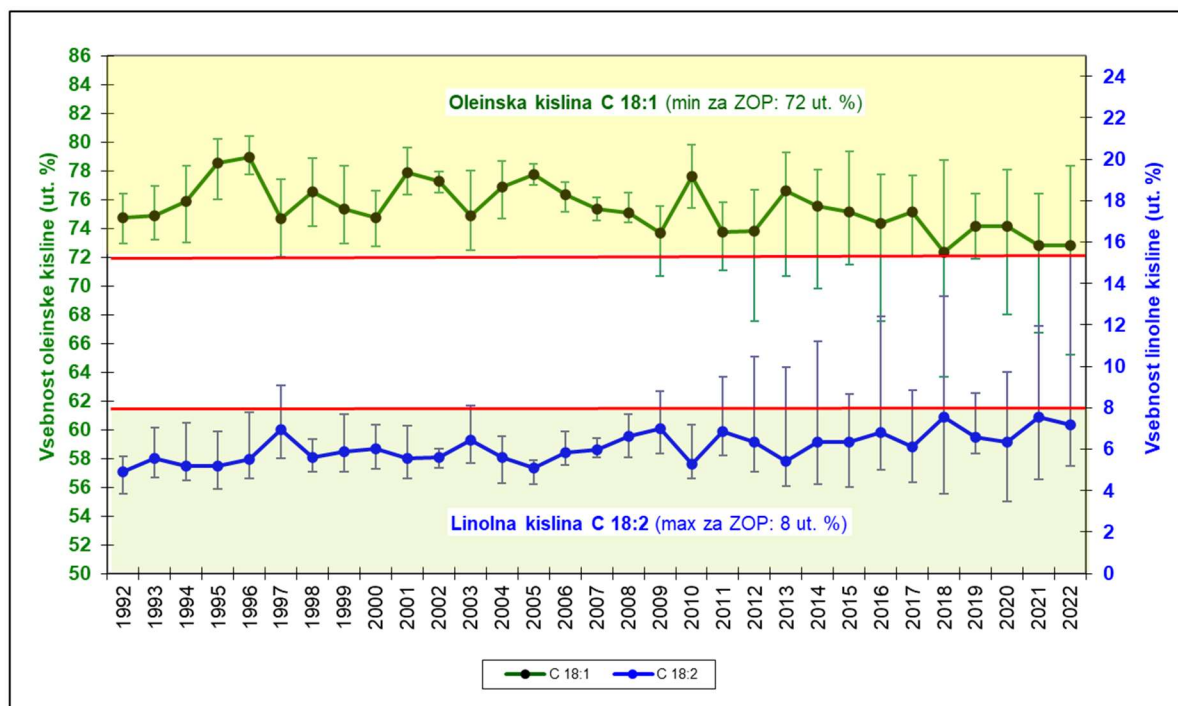
Slika 59: Vsebnost oleinske in linolne kisline v oljčnih oljih iz Slovenske Istre po posameznih letnikih. Prikazane so povprečne (zelena in modra krivulja) ter minimalne in maksimalne določene vsebnosti v posameznem letu (navpične črte).
