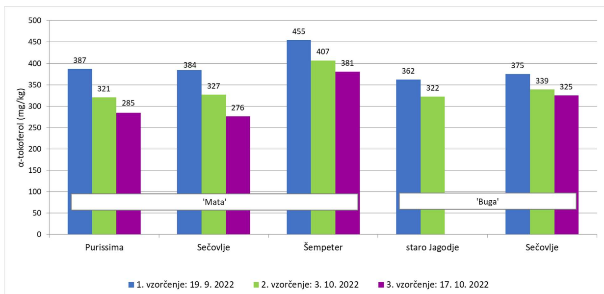
Slika 10: Vsebnost tokoferolov v oljčnih oljih iz sorte 'Mata' na lokacijah Purissima, Sečovlje in Šempeter ter sorte 'Buga' na lokacijah staro Jagodje in Sečovlje
