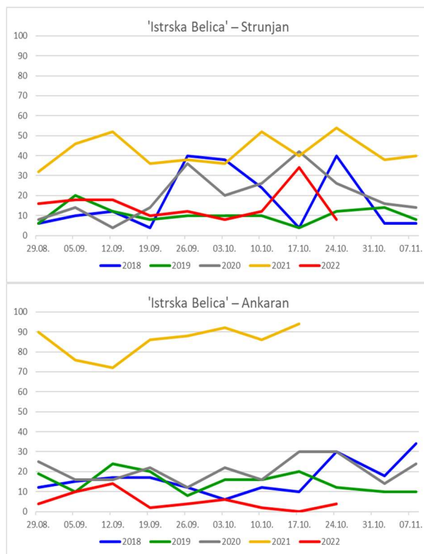
Slika 41: Odstotek poškodovanih semen v obdobju spremljanja dozorevanja pri sortah 'Istrska Belica' in 'Leccino' iz nasadov Strunjan in Ankaran v letih od 2018 do 2022
