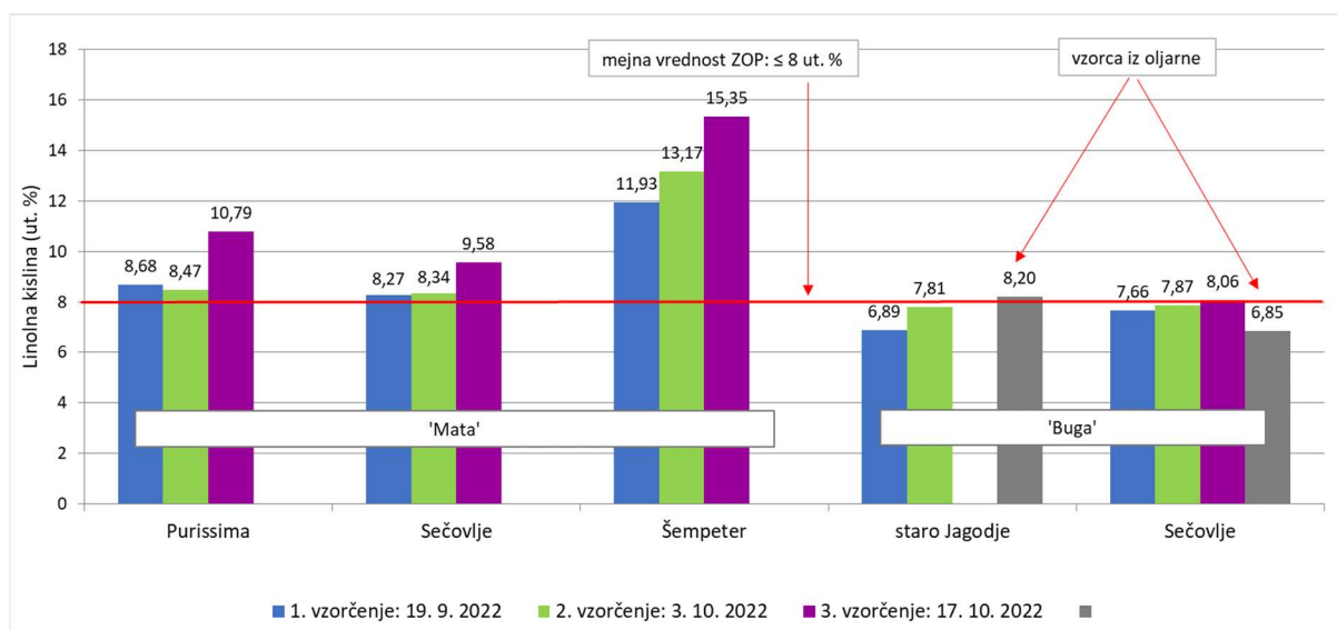
Slika 5: Vsebnost linolne kisline v oljčnem olju sorte 'Mata' na lokacijah Purissima, Sečovlje in Šempeter ter sorte 'Buga' na lokacijah Jagodje in Sečovlje
