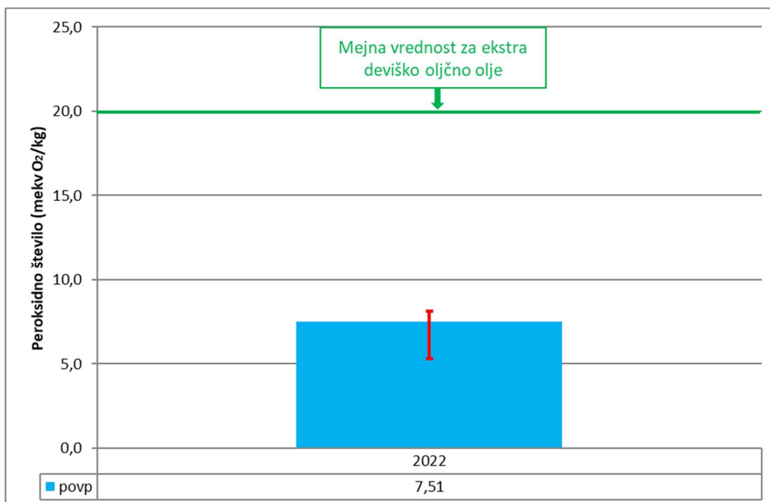
Slika 53: Določitev peroksidnega števila z metodo NIR – bližnje infrardeče spektroskopije. Modri stolpec prikazuje povprečno peroksidno število 155 vzorcev letnika 2022, z rdečo črto pa je prikazano minimalno in maksimalno peroksidno število v letniku 2022.
