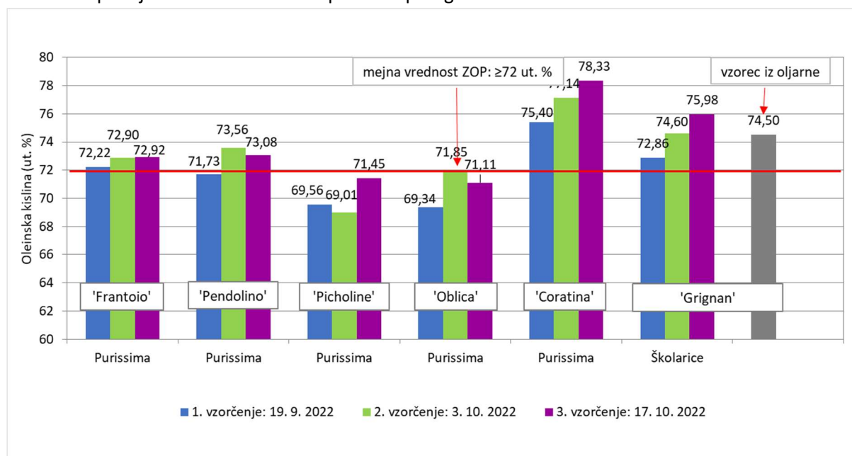
Slika 28: Vsebnost oleinske kisline v oljčnem olju sort 'Frantoio', 'Pendolino', 'Picholine', 'Oblica', 'Coratina' na lokaciji Purissima in sorte 'Grignan' na lokaciji Školarice; oljke so bile obrane v treh terminih vzorčenja, za vzorec iz oljarne pa 5. 10. 2022.
