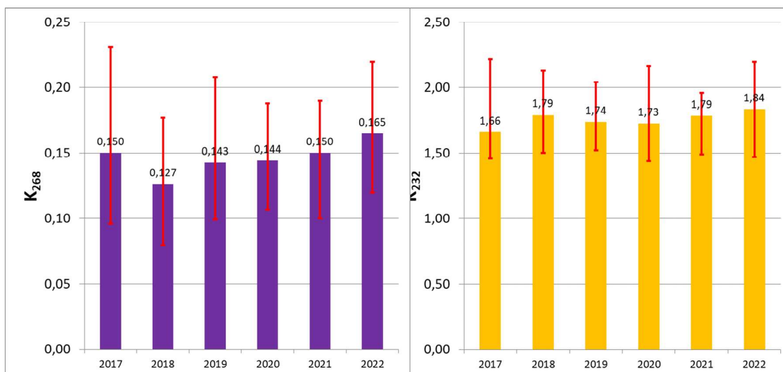
Slika 55: Primerjava parametrov K_{232} in K_{268} v 30 vzorcih letnikov 2017–2022. Stolpci predstavljajo povprečne vrednosti, z rdečo črto pa so prikazane najvišje in najnižje določene vrednosti v posameznem letu.
