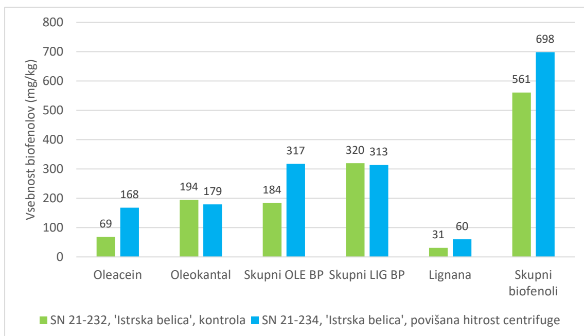
Slika 2: Primerjava vsebnosti biofenolov v olju, pridelanem s povečano hitrostjo dekanterja
