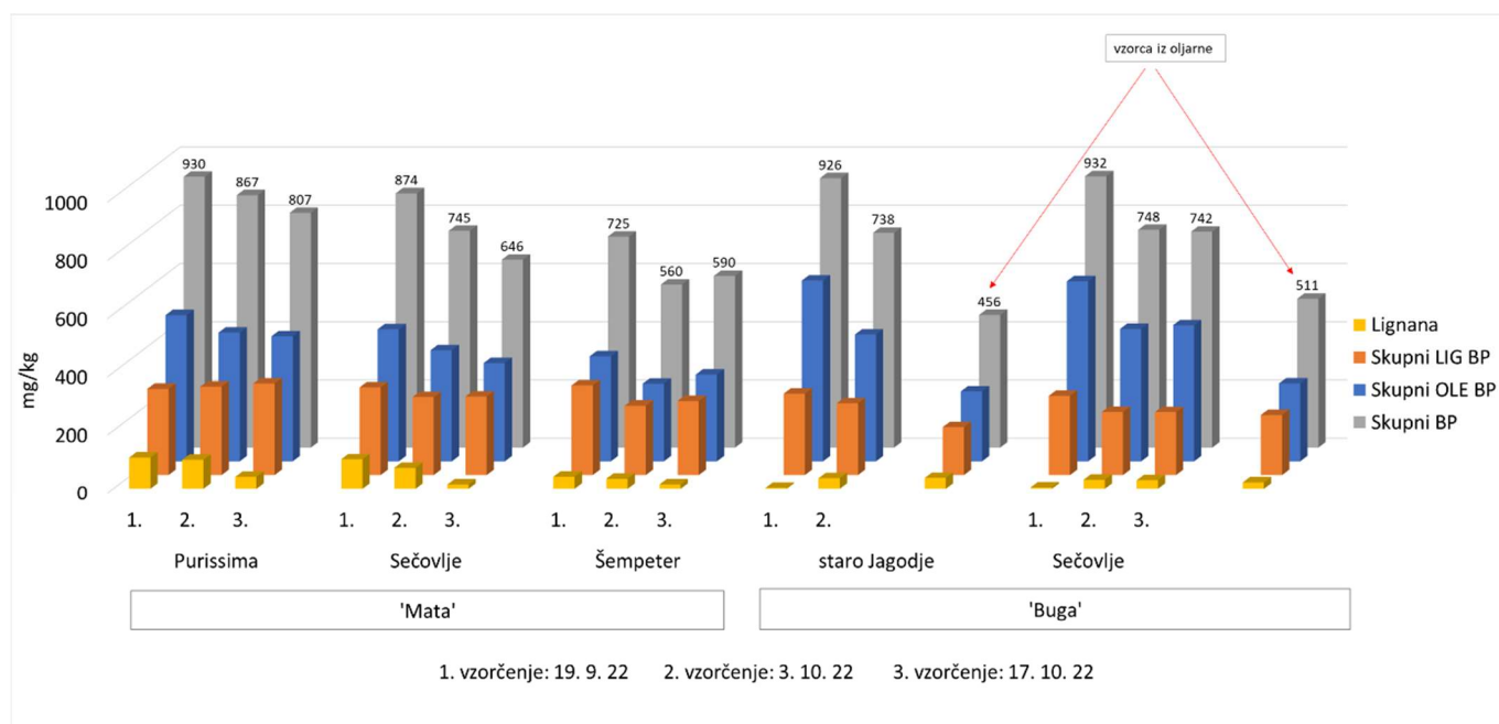
Slika 7: Primerjava vsebnosti lignanov, biofenolov ligstrozidnega (skupni LIG BP) in olevropejskega izvora (skupni OLE BP) ter skupnih biofenolov v oljčnih oljih iz sort 'Mata' na lokacijah Purissima, Sečovlje in Šempeter ter sorte 'Buga' na lokacijah staro Jagodje in Sečovlje
