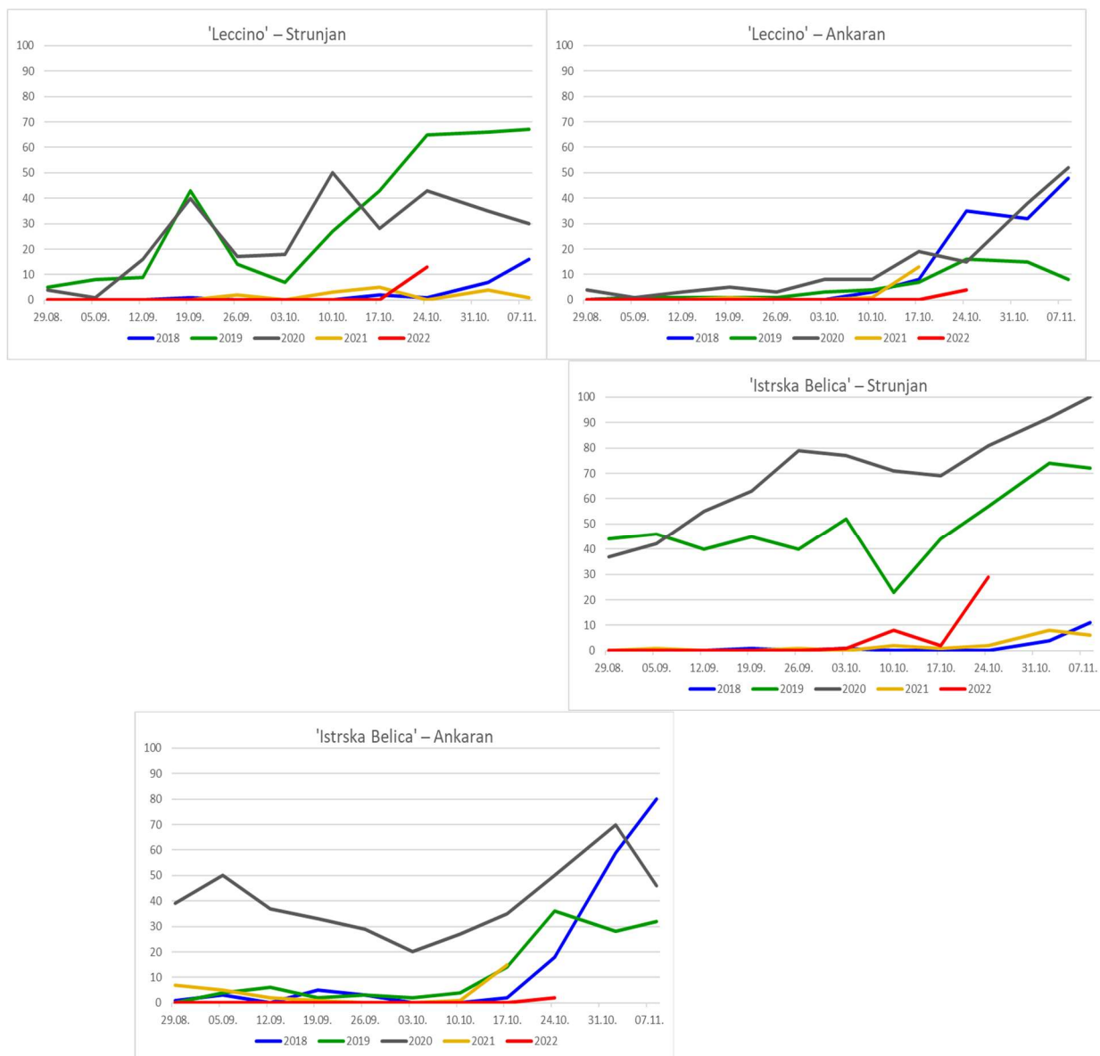
Slika 42: Odstotek poškodovanih plodov z oljno muho (izhodne luknje) v obdobju spremljanja dozorevanja pri sortah 'Istrska Belica' in 'Leccino' iz nasadov Strunjan in Ankaran v letih od 2018 do 2022
