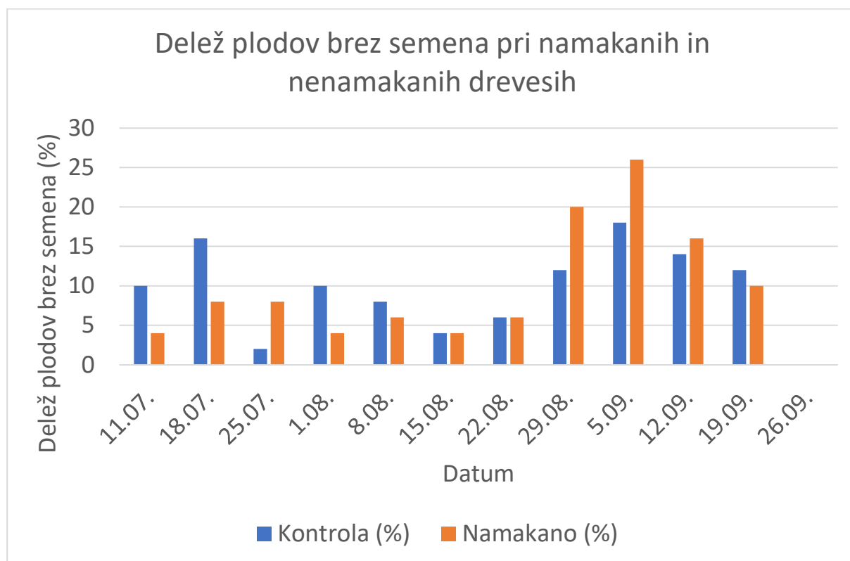
Slika 22: Povprečni delež plodov brez razvitega embrija v letu 2022 na lokaciji Semedela na sorti 'Istrska Belica'
