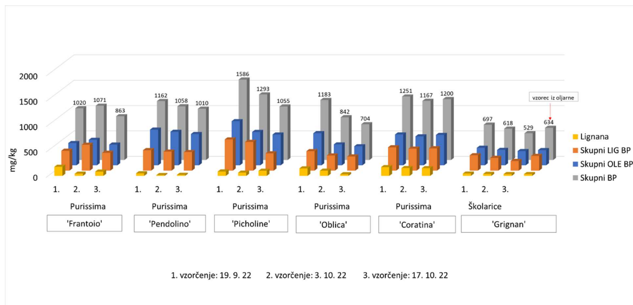
Slika 31: Primerjava vsebnosti lignanov, biofenolov ligostrozidnega (skupni LIG BP) in olevropeinskega izvora (skupni OLE BP) in skupnih biofenolov v oljčnih oljih iz sort 'Frantoio', 'Pendolino', 'Picholine', 'Oblica', 'Coratina' na lokaciji Purissima ter 'Grignan' na lokaciji Školarice; oljke so bile obrane v treh terminih vzorčenja, za vzorec iz oljarnice pa 5. 10. 2022.
