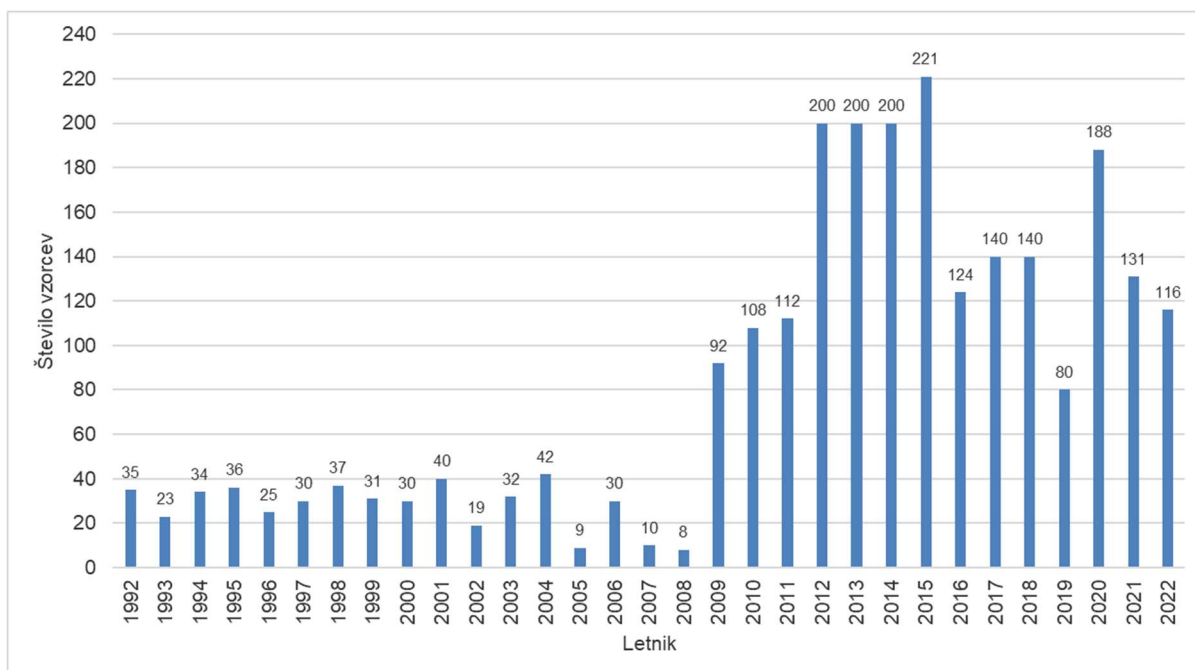
Slika 60: Število analiziranih vzorcev za določitev maščobnokislinske sestave v oljčnih oljih iz Slovenske Istre po posameznih letnikih
