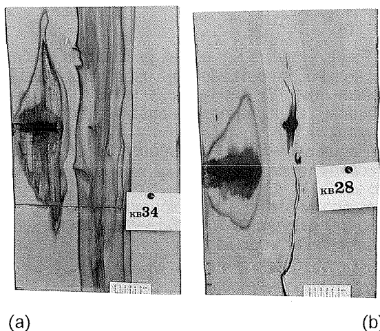
Slika 5: Bukev ( Fagus sylvatica L.): učinek globinskih poškodb, nastalih z vrtnjem v vlažno beljavo, v radialno aksialni-ravnini na primeru, kjer je poškodba neuspešno omejena (a) in obratno (b).
