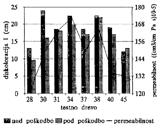
Slika 4: Bukev ( Fagus sylvatica L.), 12 testnih dreves: dolžina diskoloracij (cm), nastalih zaradi vrtanja v vlažno beljavo, merjenih v radialno-aksialni ravnini nad poškodbo in pod njo ter aksialna zračna permeabilnost.
