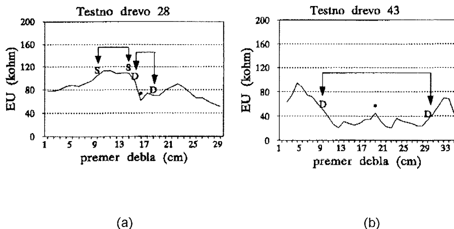
Slika 7: Bukev ( Fagus sylvatica L.): profila vertikalne električne upornosti (EU) na višini poškodb (1.3 m). V primeru (a) je še prisoten del primarno nastale sušine, v primeru (b) je diskoloriran celoten centralni del debla.
