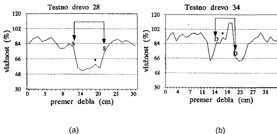
Slika 6: Bukev ( Fagus sylvatica L.): vlažnostna profila na višini 1.05 m: (a) padec vlažnosti proti strženu zaradi naravnega fiziološkega izsuševanja sredice in (b) sekundarni dvig vlažnosti na poprej nastali sušini zaradi diskoloracije lesa po ranitvi.
