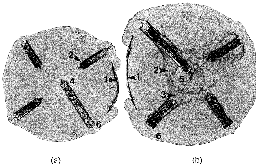
Slika 2: Bukev ( Fagus sylvatica L.): učinek poškodb na prečnem prerezu debla na primeru, ko so učinki poškodovanja uspešno omejeni (a) in obratno (b).
