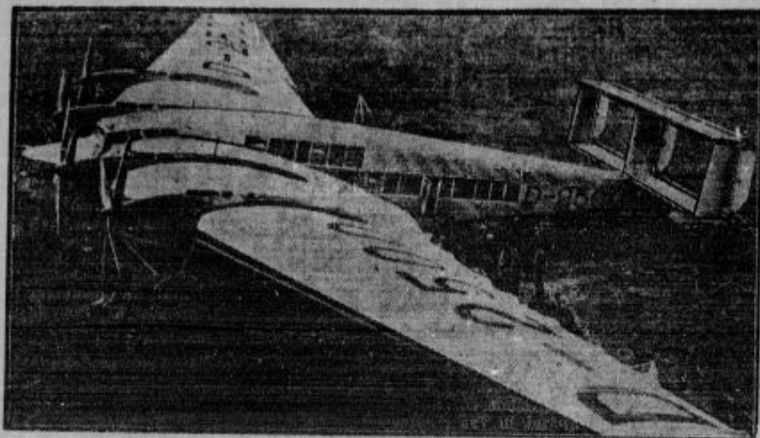
24.000 kg teško Junkersovo letalo »D 2500«.
