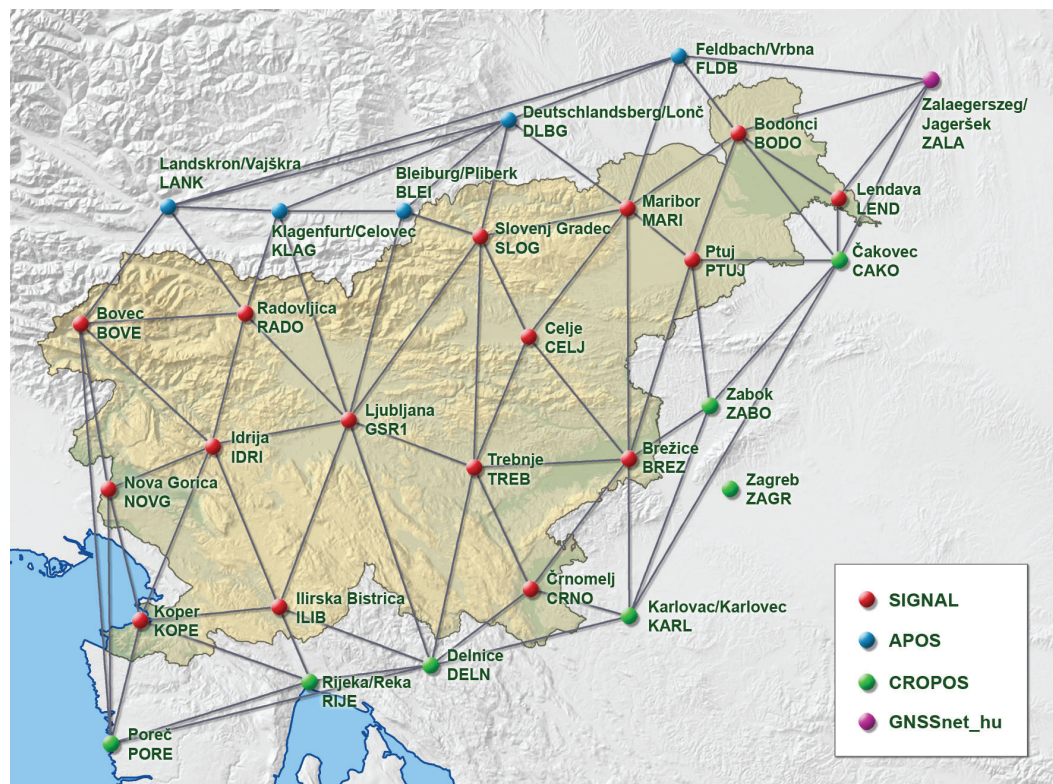
Slika 1: Skica omrežja stalnih postaj SIGNAL.
