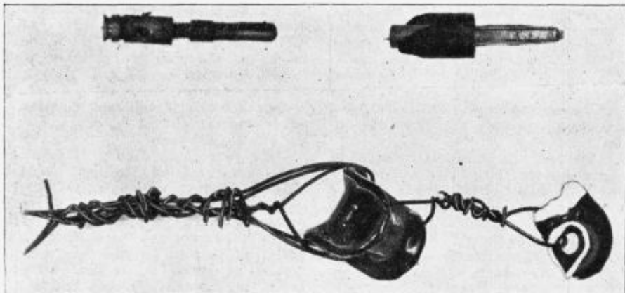
Od strele v radioaparatu obžgane banane in skvarjeni antenski izolatorji.
