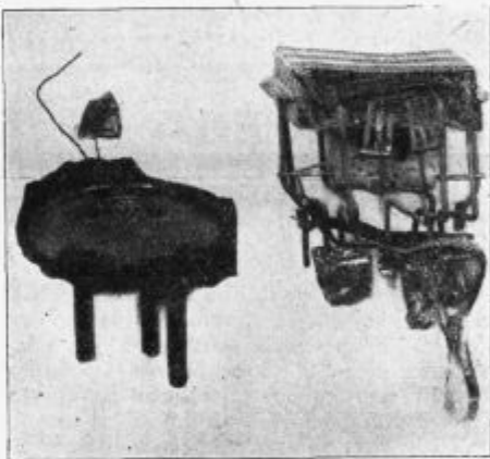
Razvaline Philipsove elektronke v aparatu, v katerega je udarila strela.
