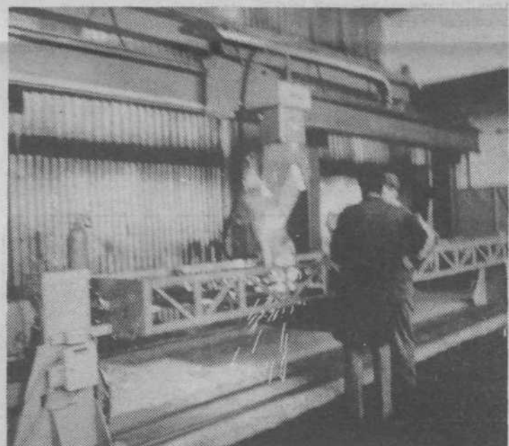
Takšen je videti robot za varjenje (Foto: D. J.)
