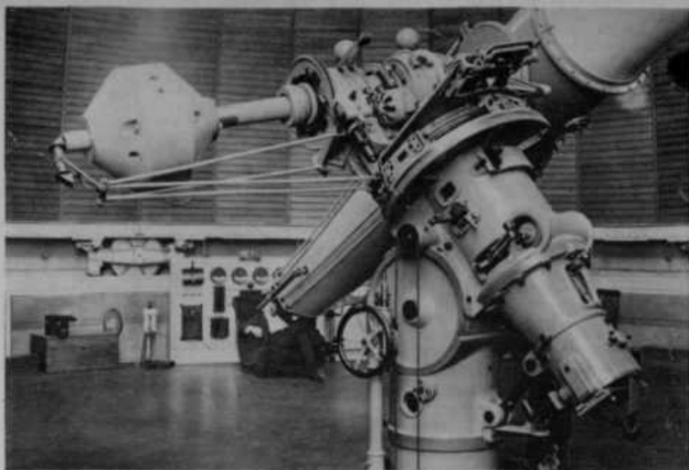
Ogromni daljnogled v berlinski zvezdarni. S tem daljnogledom opazujejo solčne mrke in premikanje vseh nebesnih teles kar najatančneje.
