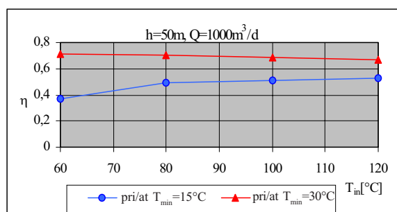
Sl. 4. Izkoristek sistema kot funkcija temperature vode pri polnjenju T_{\text{in}} , T_{\min}=30^{\circ}\text{C} in T_{\min}=15^{\circ}\text{C}
