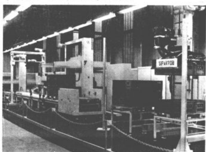
Nov stroj — Sipak rob predstavlja skupaj s povezovalno nakladalno razkladalno linijo povsem avtomatiziran proces pakiranja, nakladanja oziroma razkladanja izdelkov. S tem je odpravljeno ozko grlo v proizvodnji pri pakiranju.
