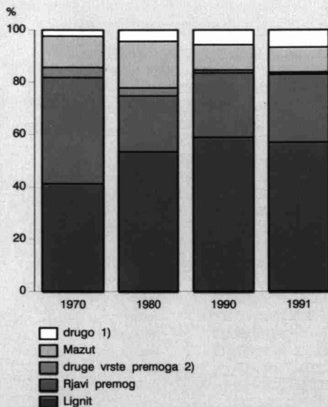
STRUKTURA EMISIJ ŽVEPLOVEGA DIOKSIDA PO NOSIL- CIH ENERGIJE, 1970, 1980, 1990, 1991
