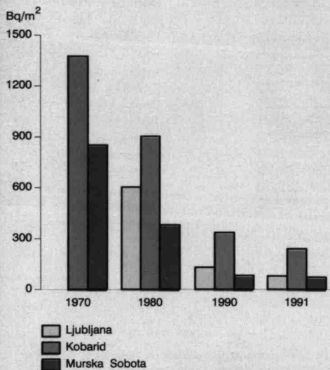
POVPREČNA LETNA SPECIFIČNA AKTIVNOST STRONCI- JA - 90 V VZORCIH ZEMLJE V GLOBINI OD 0 DO 5 CM, 1970, 1980, 1990, 1991
