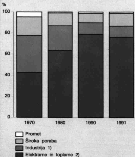
STRUKTURA EMISIJ ŽVEPLOVEGA DIOKSIDA PO PORAB- NIKIH GORIV IN SUROVIN, 1970, 1980, 1990, 1991
