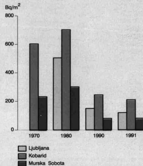
POVPREČNA LETNA SPECIFIČNA AKTIVNOST STRONCIJA - 90 V VZORCIH ZEMLJE V GLOBINI OD 10 DO 15 CM, 1970, 1980, 1990, 1991
