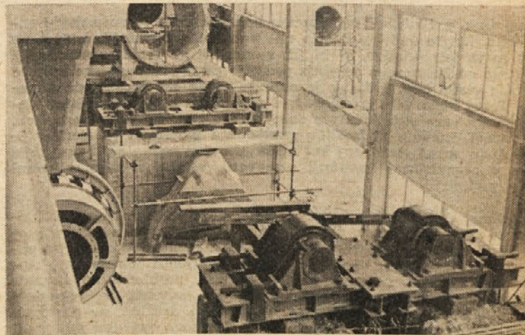
Pred dnevi so naši vzdrževalci dokončali veliko delo — zaključili so remont v obratu litopona. Na sliki: zgoraj: nove »rolke« na katerih se že vrtili nova rotacijska peč. Na sliki spodaj: vzdrževalci popravljajo filterske stiskalnice
