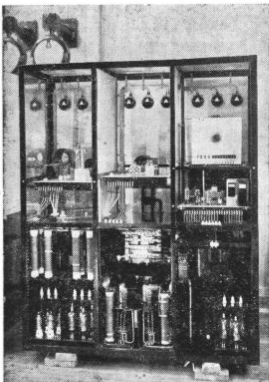
Na sliki vidimo v aluminijastih omarah montirane pentodne stopnje I.—IV. Ker prenovitev še ni popolnoma dovršena, se vidijo na slikah poleg nove aparature tudi deli stare aparature iz l. 1918.
