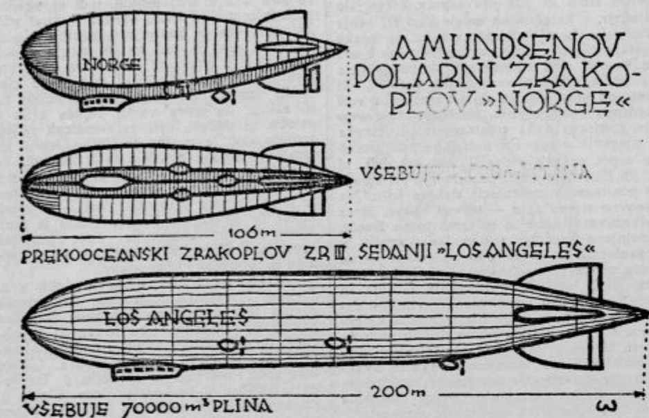
Ameriška zračna križarka »Los Angeles« v primeri z »Norge«
