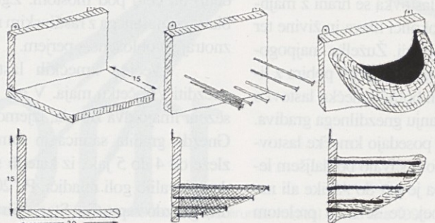
Načrti za izdelavo gnezdilnih polic Risba: S. Polak
