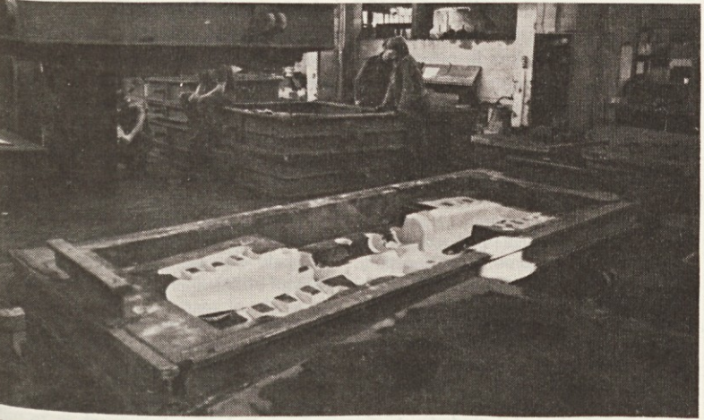
Spodnji del forme za člen bagske gosenice rudniškega bagra namenjena za dnevni kop (Foto: T. Š.)
