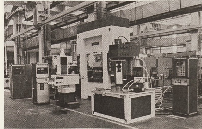
Fleksibilna preoblikovalna celica FPC-400-HSO-2-160
