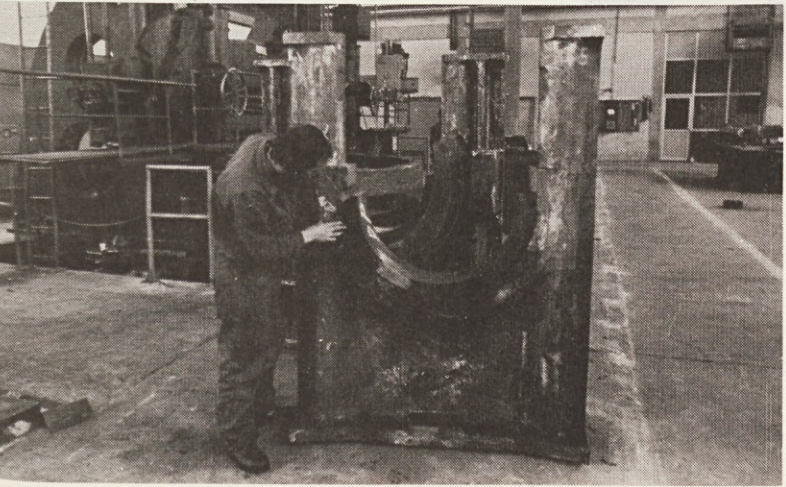
Jekleni ulitki nosilnih ležajev za ladijske motorje (Foto: T. Š.)
