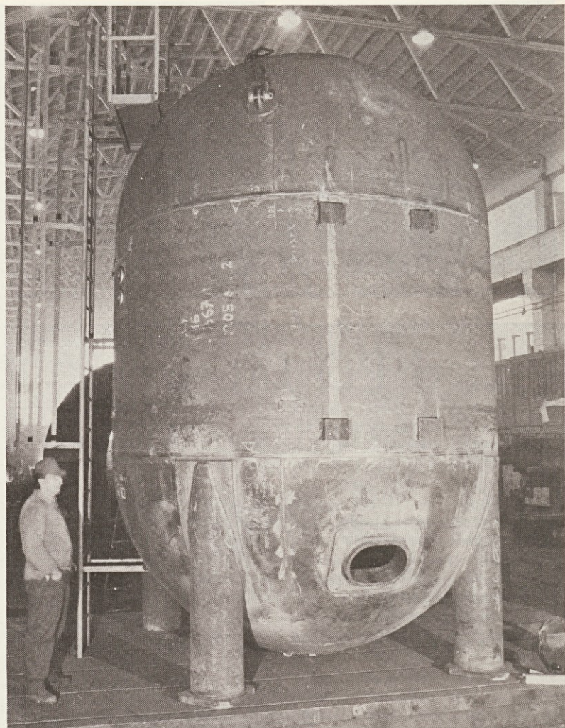
Tlačni kotel za ČP Kirkuk s prostornino 40 m 3 in težo 9.800 kg za razbremenitev tlačnega cevovoda. Posebnost tovrstnega kotla so polkroglaste podnice sestavljene iz šestih segmentov. Problem polkroglaste smo uspešno rešili v sodelovanju med tozdom PZO in obrtnikom inženirjem Terlepom, ki je segmente prostorsko ukrivil.
