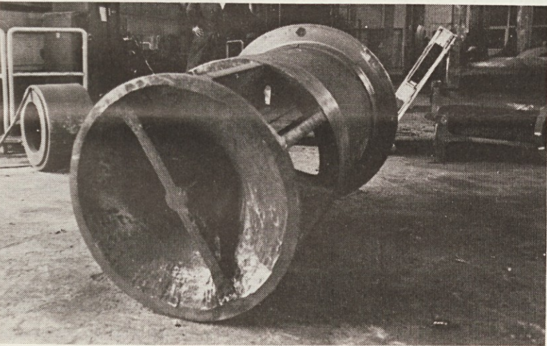
Ulitek vstopnega grla za rudniške naprave na finem čiščenju v čistilnici jeklolivarne (Foto: T. Š.)
