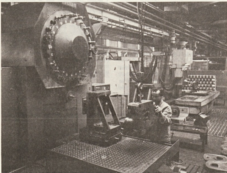
V tozdu TVN so na numerično krmiljenem stroju EX-CELL-O končali z izdelovanjem glav cilindrov T 23 L-2 za dizelske motorje. To delo je trajalo dva meseca, proti koncu pa so delali noč in dan, ker se je že zelo mudilo. Tovrstnega dela v tozdu Obdelava ne morejo narediti sami, ker nimajo ustreznih strojev, v tozdu TVN pa za proizvodnjo dizelskih motorjev izdelujejo še precej drugih delov. (Foto: T. Š.)
