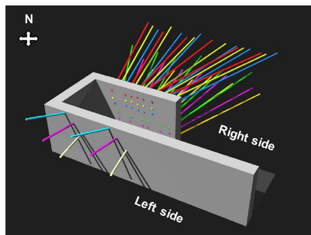
Fig. 2. Scheme of the lysimeter construction. Sl. 2. Shema kostrukcije lizimetra.
