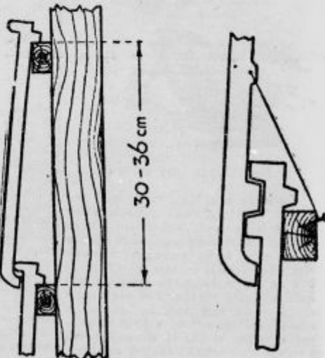
Sl. 10. Izvedba kritja s strešniki.
