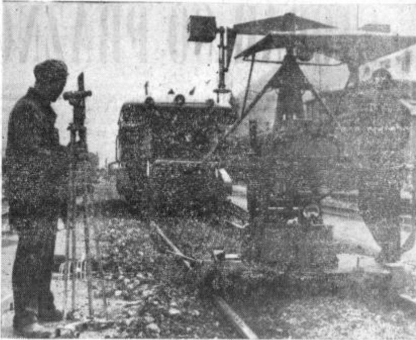
Posnetek prikazuje nov podbitalni stroj pri utrjevalnih delih na celjski železniški postaji.
