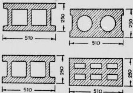
Sl. 3. Najobičajnejše oblike betonskih votlakov ali klad.
