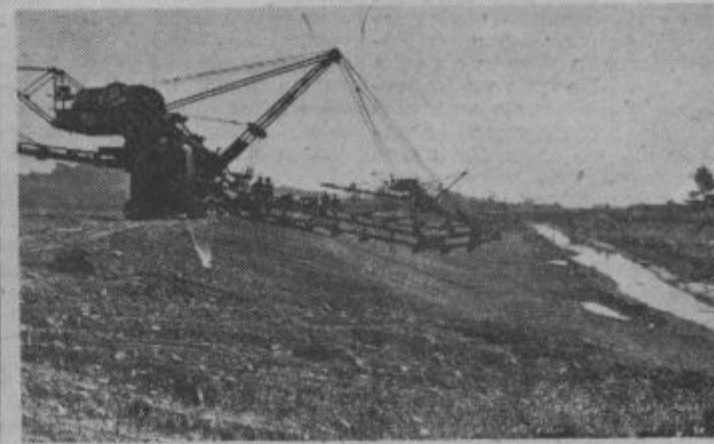
Zemeljska dela na odvodnem kanalu blizu naselja 5D 1, na delovnišču »Tehnoigradenj«.
