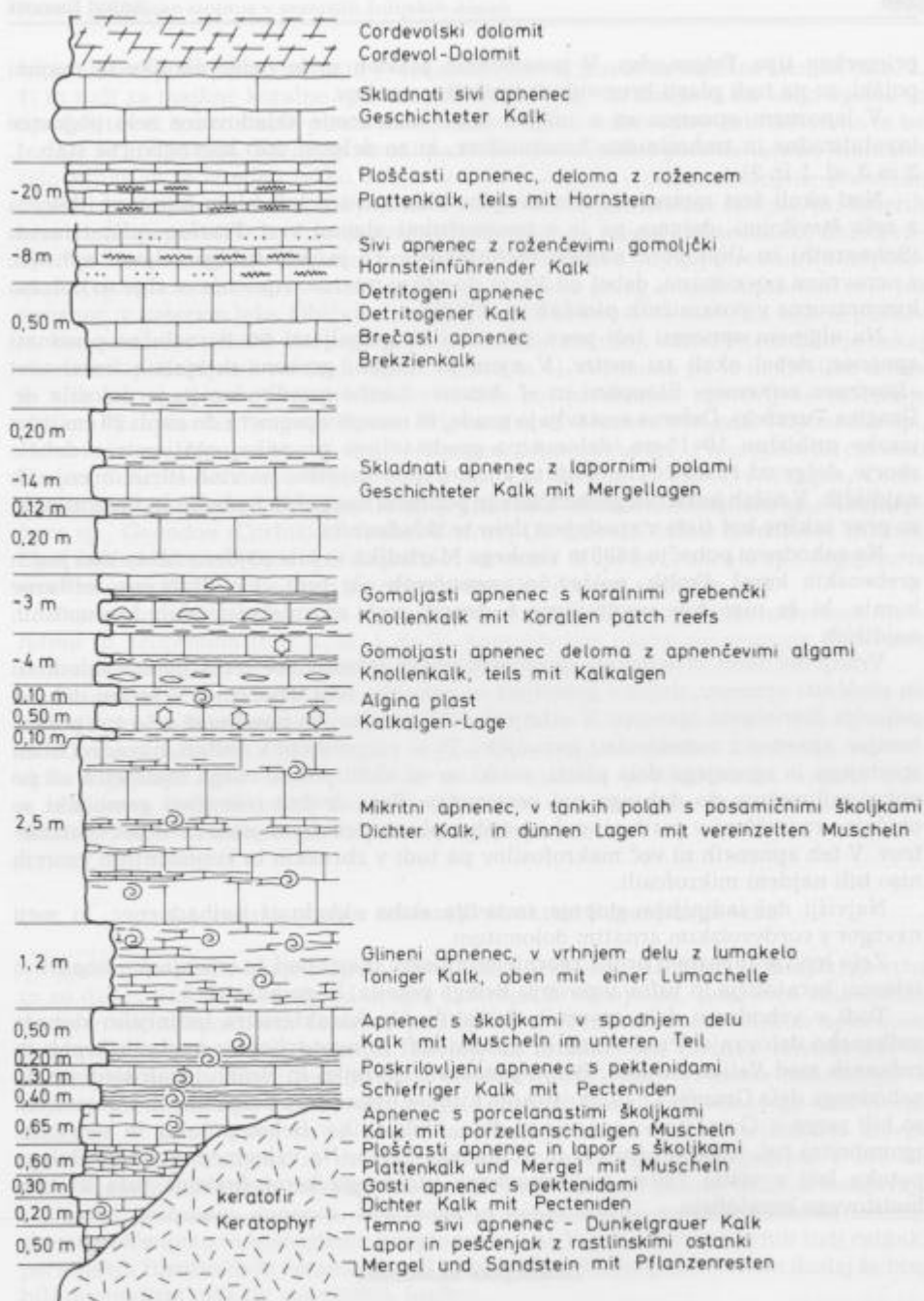
Sl. 3. Stratigrafska lestvica zgornjega ladinjskega horizonta na ozemlju Belega potoka
