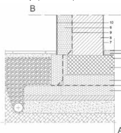
Primer ustrezne izvedbe stika stene s temeljno ploščo (VIR)
