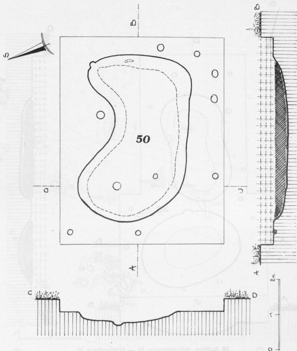
11 Jazbine: poluzemunica 50 — Grubenhaus 50
