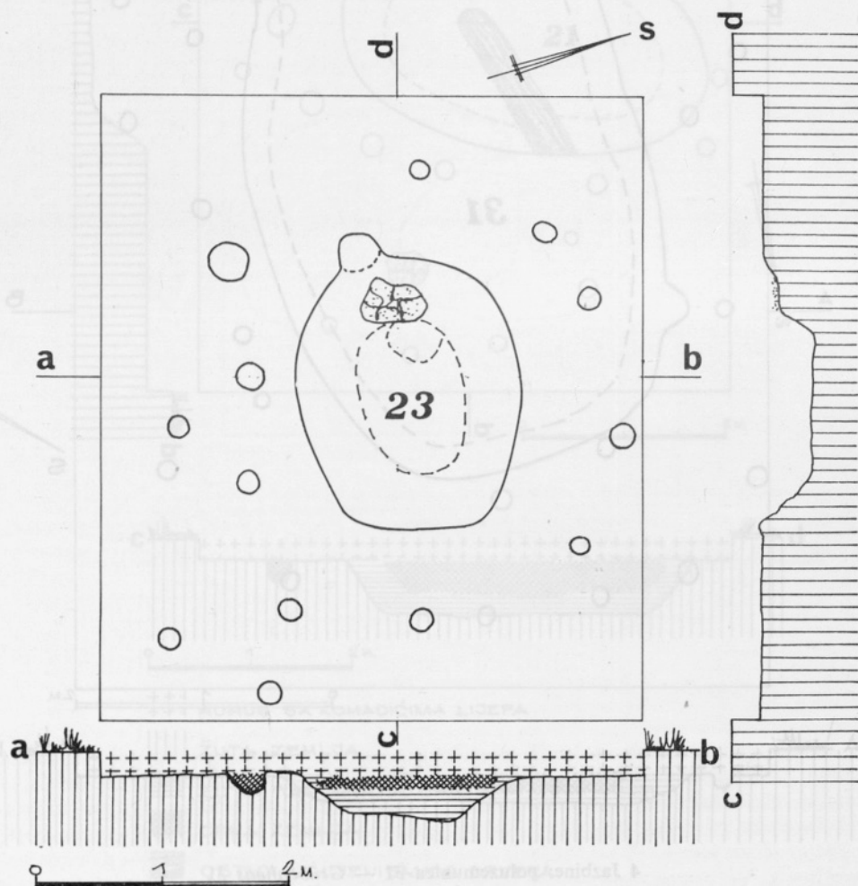
5 Jazbine: poluzemunica 23 — Grubenhaus 23
