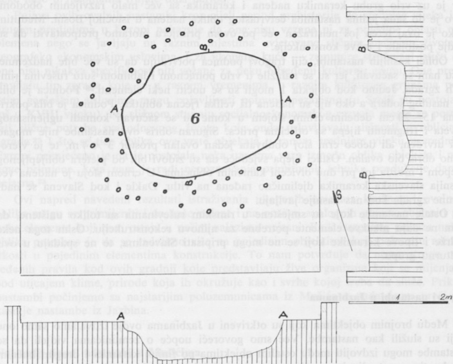
1 Jazbine: poluzemunica 6 — Grubenhaus 6
