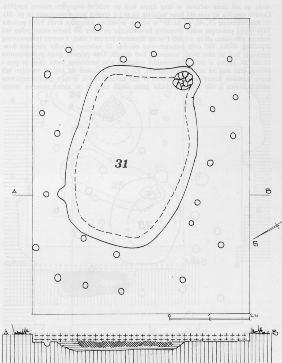
4 Jazbine: poluzemunica 31 — Grubenhaus 31
