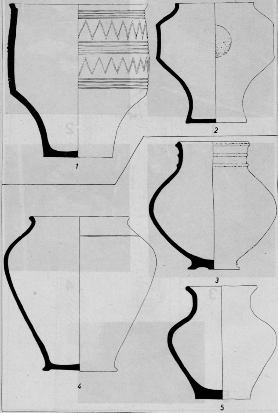
Sl. 1, 2 in 4 = \frac{1}{2} , sl. 3 in 5 = \frac{1}{4} n. vel.
