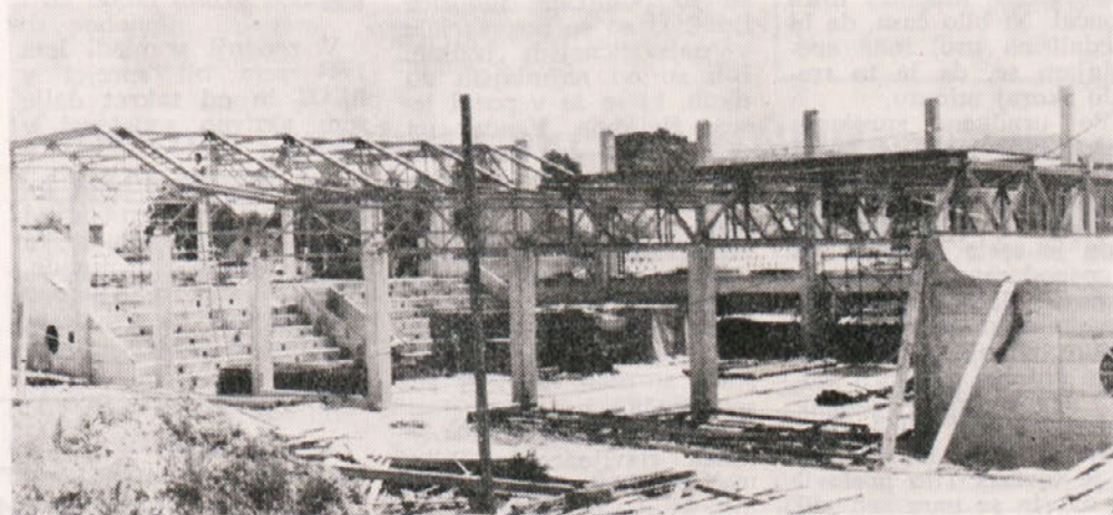
Na gradbišču SRC Golovec montaža strešne konstrukcije nad kegljiščem in bazenom
