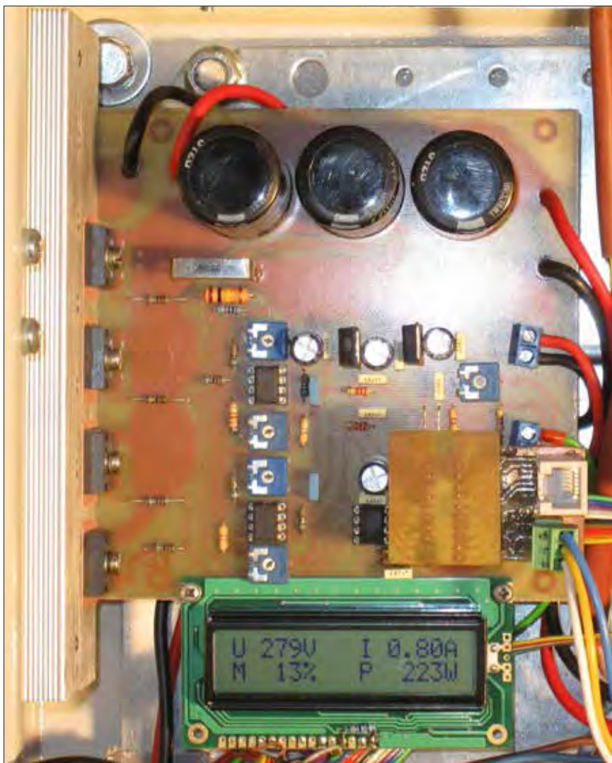
Slika 5. Vezje MPP-sledilnika
