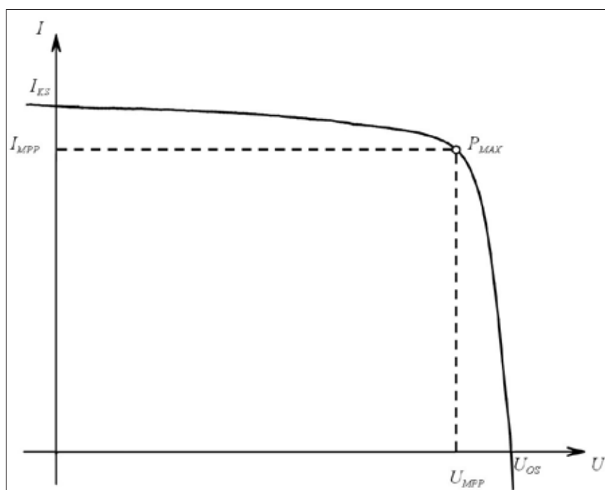
Slika 2. Graf U-I sončne celice z označeno točko maksimalne moči
