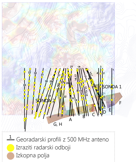
15 Položaj georadarskih profilov s 500 MHz anteno in izraziti radarski odboji, ki so bili izmerjeni vzdolž teh profilov; M 1:1000.
