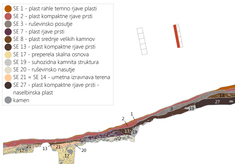
21 Čateški grič – sondiranje 2000 (Čateški grič I), sonda 1, zahodni profil; M 1 : 100.
