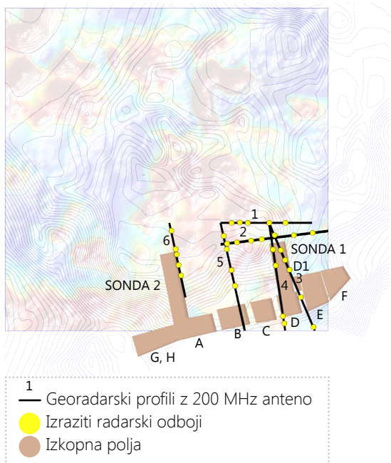
14 Položaj georadarskih profilov z 200 MHz anteno in izraziti radarski odboji, ki so bili izmerjeni vzdolž teh profilov; M 1:1000.
