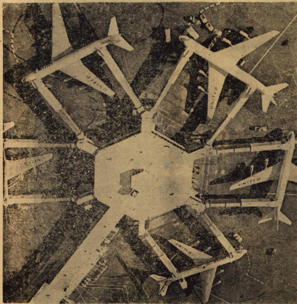
Pristajališčna zgradba letališča v San Franciscu ima obliko zobčenika. Premični pokriti prehodi neposredno povezujejo izhod iz letala s čakalnico. Dolžina teh prehodov se lahko menja, z njimi upravljajo s pomočjo elektromagnetov, namestiti pa jih je mogoče v manj kot 60 sekundah.
