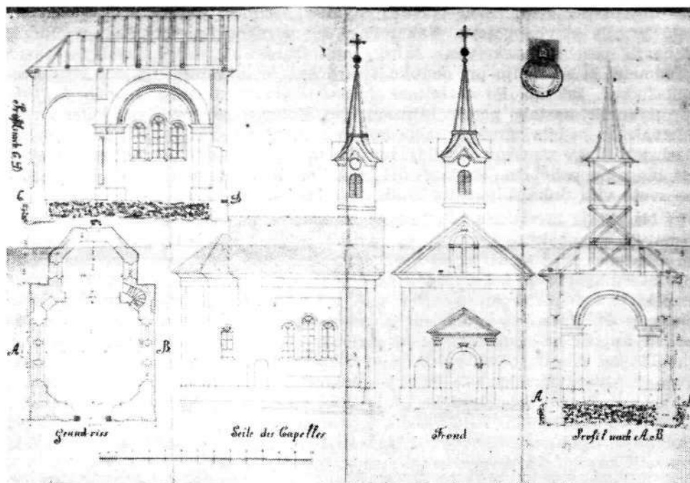
Molinarijev načrt kapele za pokopališče v Skofji Loki. (Po izvirniku v Zgodovinskem arhivu v Skofji Loki.)
