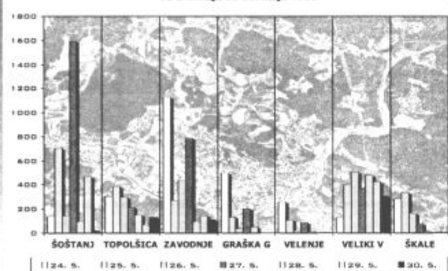
MAKSIMALNE POLURNE KONCENTRACIJE SO 2 od 24. maja do 30. maja 1999
