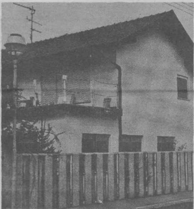
Jubizol sistem je namenjen za zunanjo toplotno izolacijo fasadnih zidov. Sestavljen je iz styropor plošč, ki so z zunanje strani zaščitene s tankim, s stekleno tkanino ojačanim osnovnim ometom (Fotoarhiv Izolirke)
