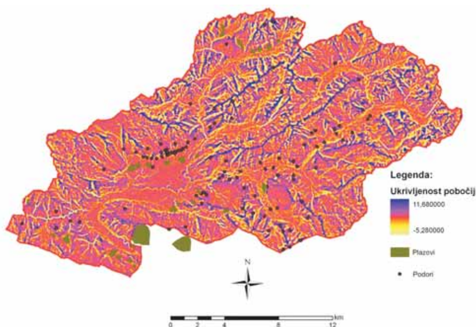
Slika 6. Karta ukrivljenosti pobočij za območje občine Bovec
