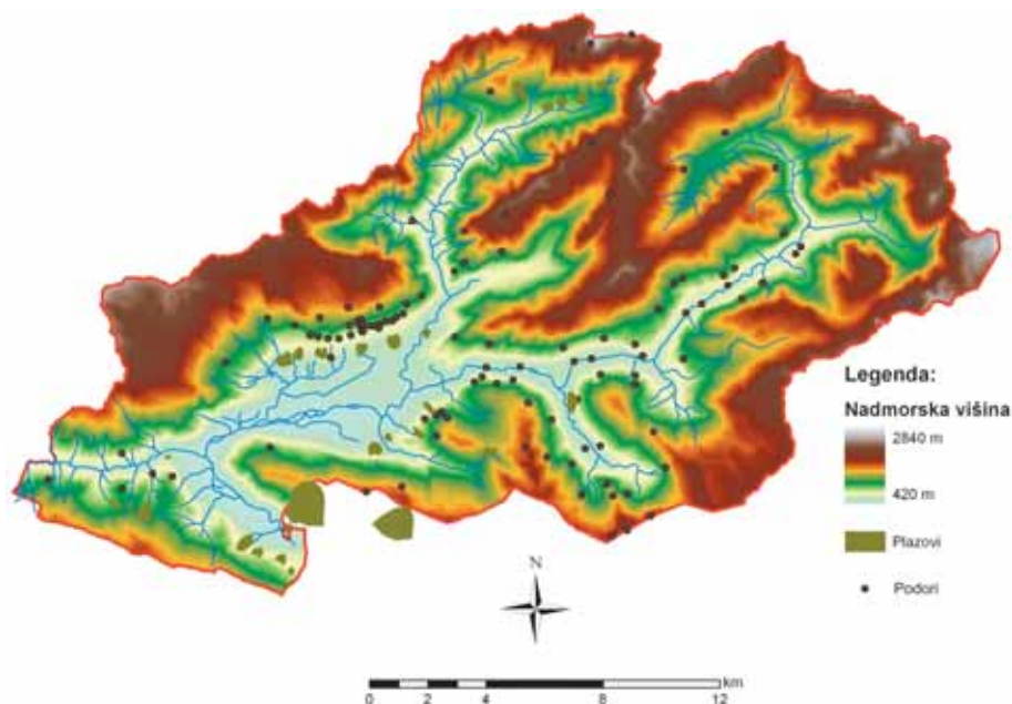
Slika 4. Karta nadmorskih višin za območje občine Bovec
