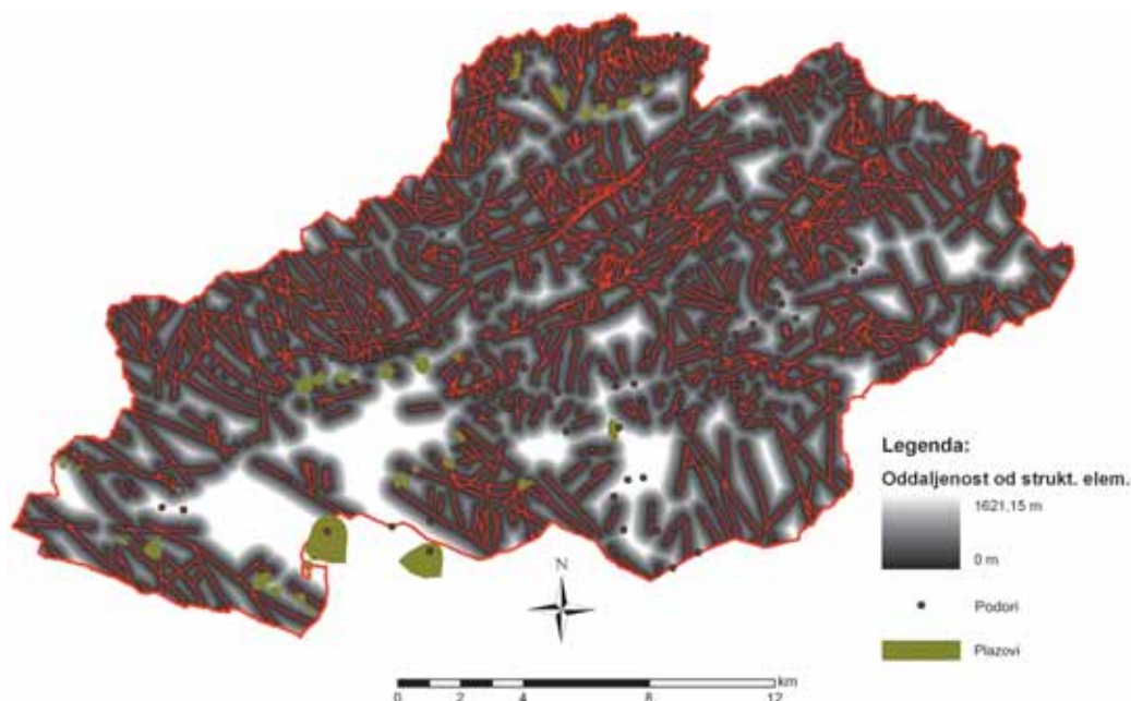
Slika 9. Karta oddaljenosti od strukturnih elementov za območje občine Bovec
