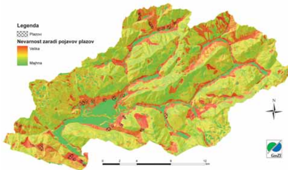
Slika 13. Verjetnostni model napovedi nevarnih območij zaradi pojavov plazov za območje občine Bovec in lokacije znanih plazov
