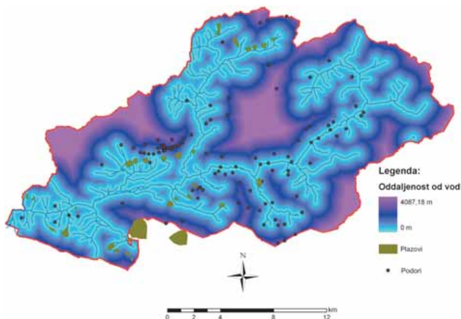
Slika 8. Karta oddaljenosti od površinskih tokov (vod) za območje občine Bovec
