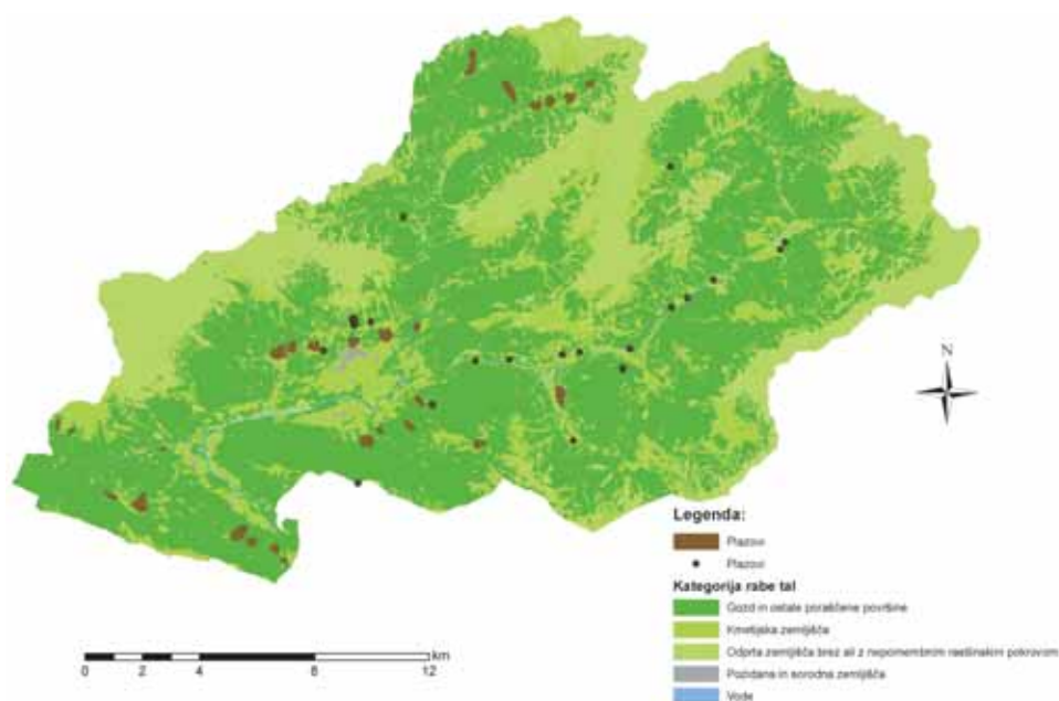
Slika 11. Karta tipov rabe tal za območje občine Bovec (MKGP, 2002)
