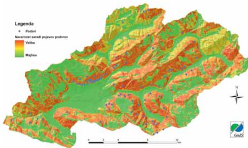
Slika 14. Verjetnostni model napovedi nevarnih območij zaradi pojavov podorov za območje občine Bovec in lokacije znanih podorov
