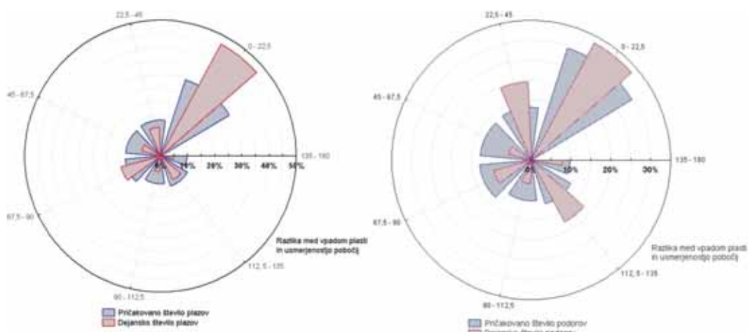
Slika 12. Rožni diagram pojavljanja plazov (levo) in podorov (desno) glede na sinhronost vpadov plasti in usmerjenost pobočij za območje občine Bovec
