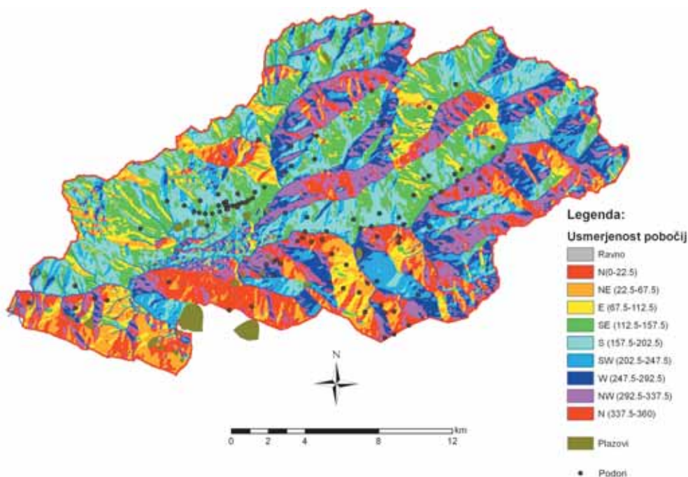
Slika 7. Karta usmerjenosti pobočij za območje občine Bovec
