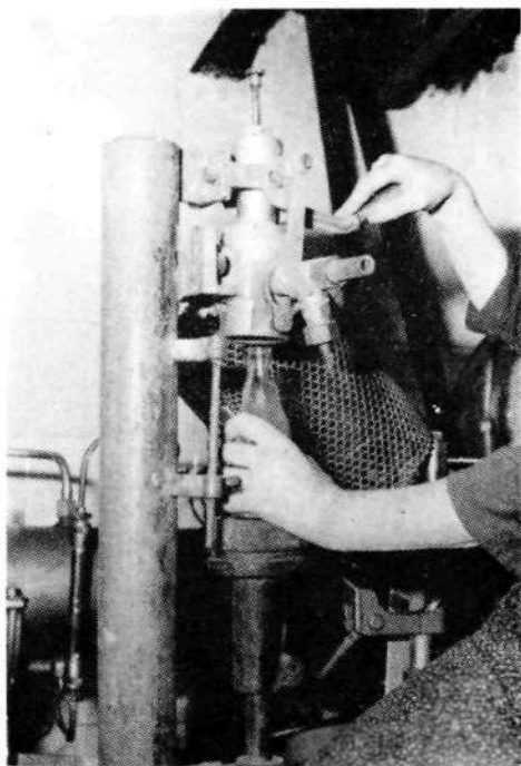
Polnilni in zapiralni stroj za »šabeso«, steklenice z aluminijastimi kapicami. Rekonstrukcija v avgustu 1984 v opuščeni delavnici pri Fušarjevih v Skofji Loki
