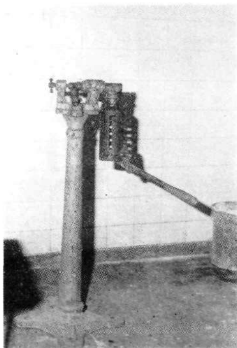
Polnilni in zapiralni stroj za pokalico, »krahrl« v opuščeni delavnici pri Fušarjevih v Skofji Loki
