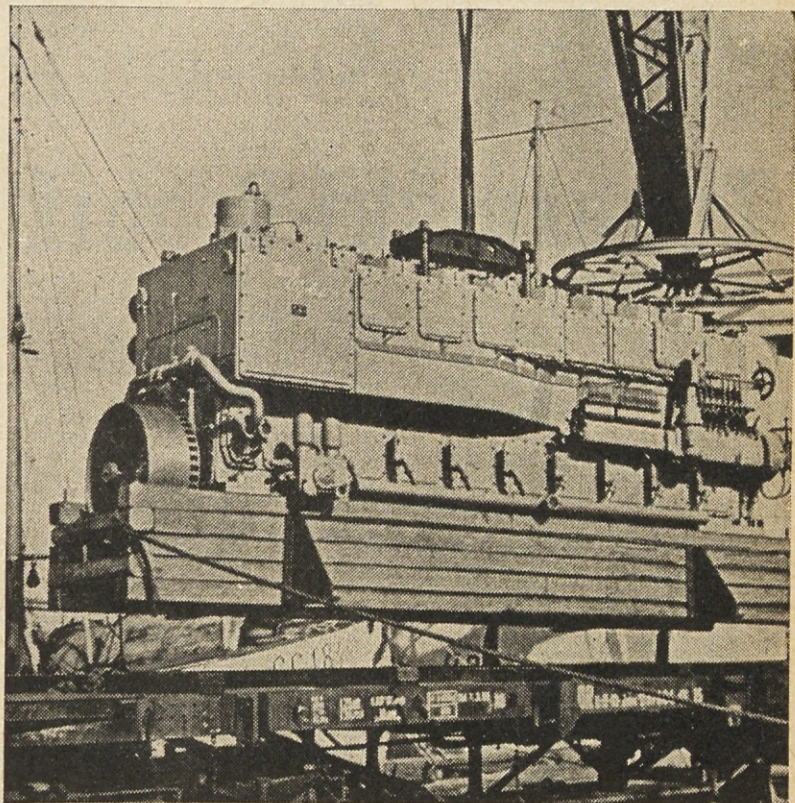
8-cilindrski ladijski diesel motor familije Alpha, tipa 490 R. Motor ima moč 960 KS pri 310 o/min. Premer cilindra 290 mm, gib bata 490 mm. V delu imamo 10 takih motorjev
