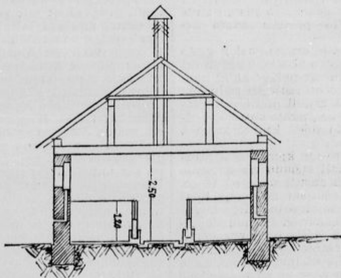
Podoba št. 3: Pošesni prerez.
