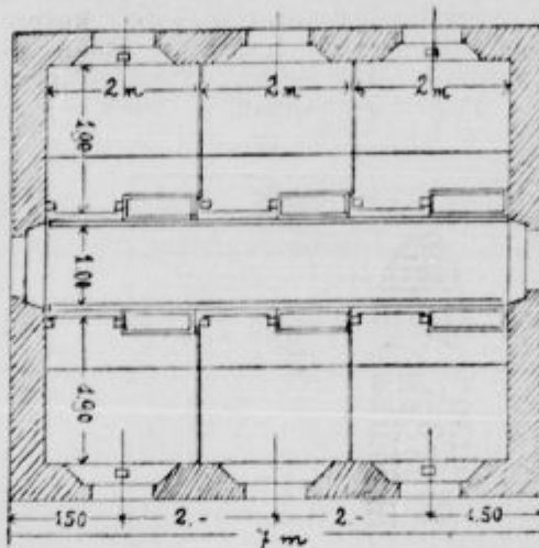
Podoba št. 1: Tloris.
