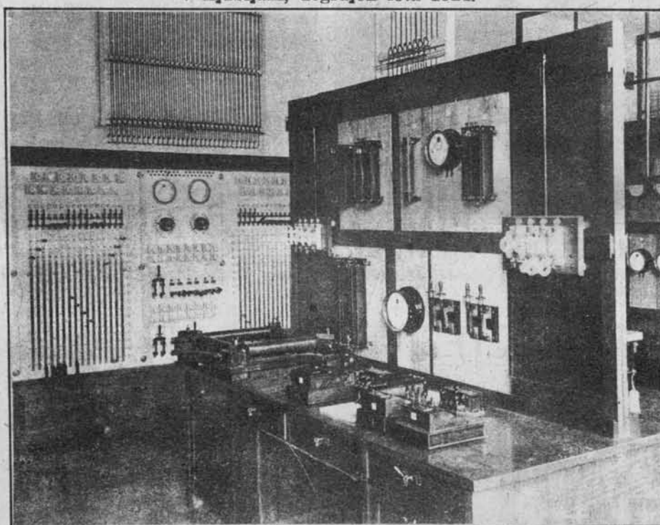
Stikalna deska z merilno mizo v slušateljskem laboratoriju elektrotehniškega instituta na slovenski univerzi v Ljubljani.
