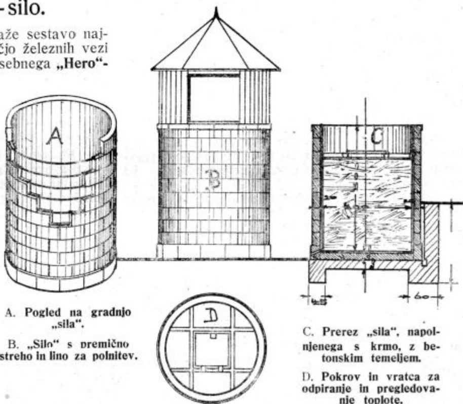
Pod. 6. Načrti najnovejšega Herba-silo.
