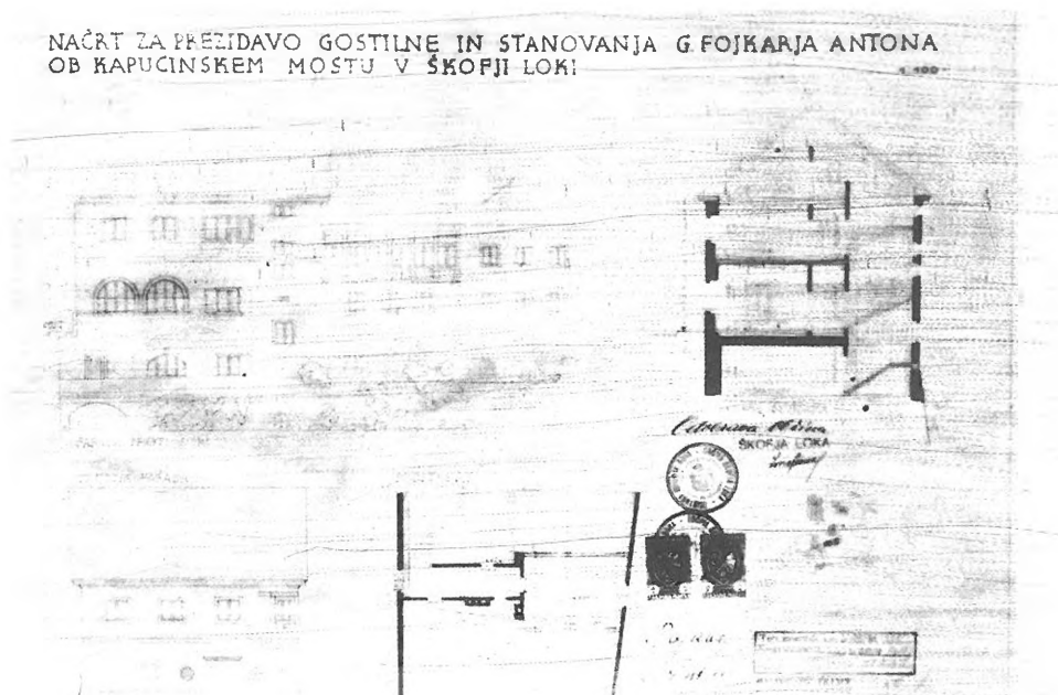
Načrti za adaptacijo hiše Kapucinsko predmestje 14, danes Titov trg 11 ob Kapucinskem mostu. Zgornji načrt je izdelal Janez Krstnik Molinaro leta 1888, spodnjega pa ing. France Tomažič iz Ljubljane leta 1938. Original ZAL Škofja Loka, foto Šturm.
