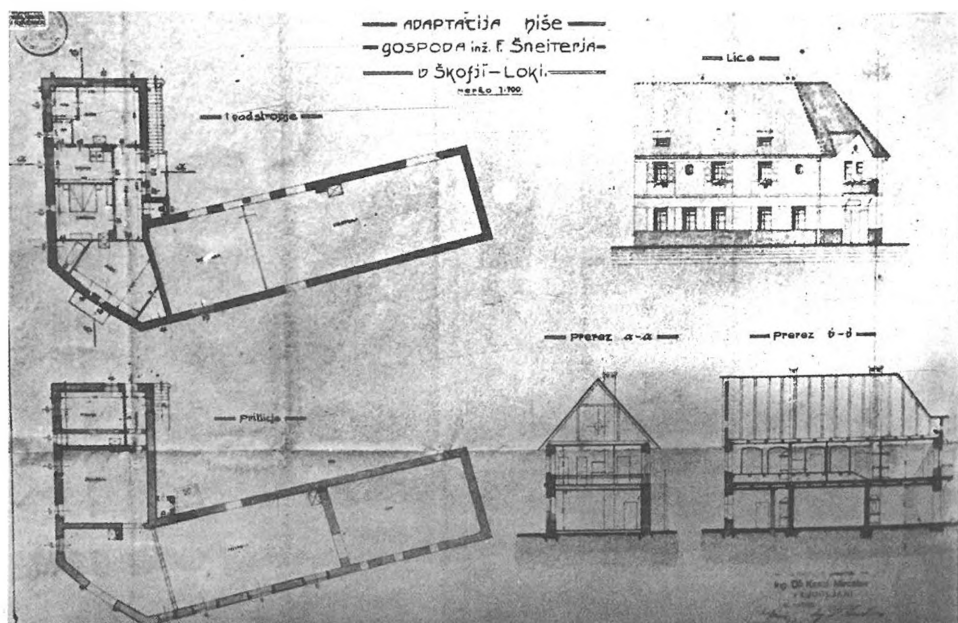
Načrti adaptacije Krennerjeve pristave na Studencu v stanovanjsko hišo in tovarno turbin ing. Franca Schneiderja, Studenec 26. Sedaj je v stavbi AMD Škofja Loka, Jegorovo predmestje 10. Načrte je izdelal ing. dr. Miroslav Kassal leta 1922. Original ZAL Škofja Loka, foto Šturm.
