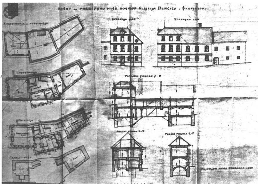
Neizvedeni načrti prizidave Jakličeve hiše, Kapucinsko predmestje 13, sedaj Titov trg 12. Načrt je bil izdelan v Ljubljani 1906.
