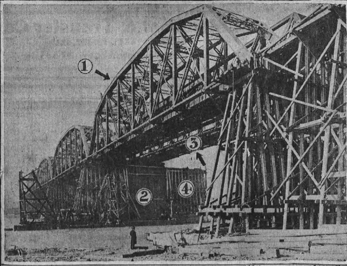
NOVI IN STARI ŽELEZNIŠKI MOST ČEZ REKO MISSOURI V OMAHI.
