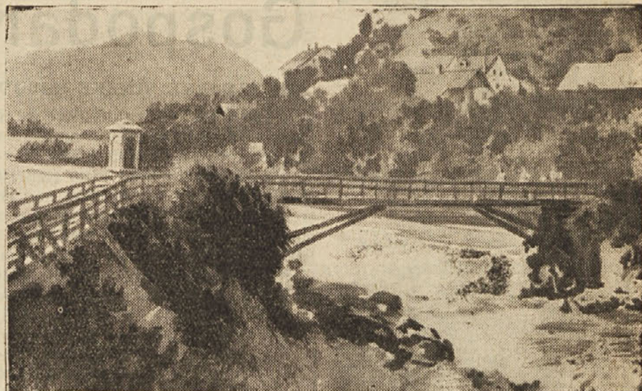
Puštalska brv v Škofji Loki pred poplavo.
