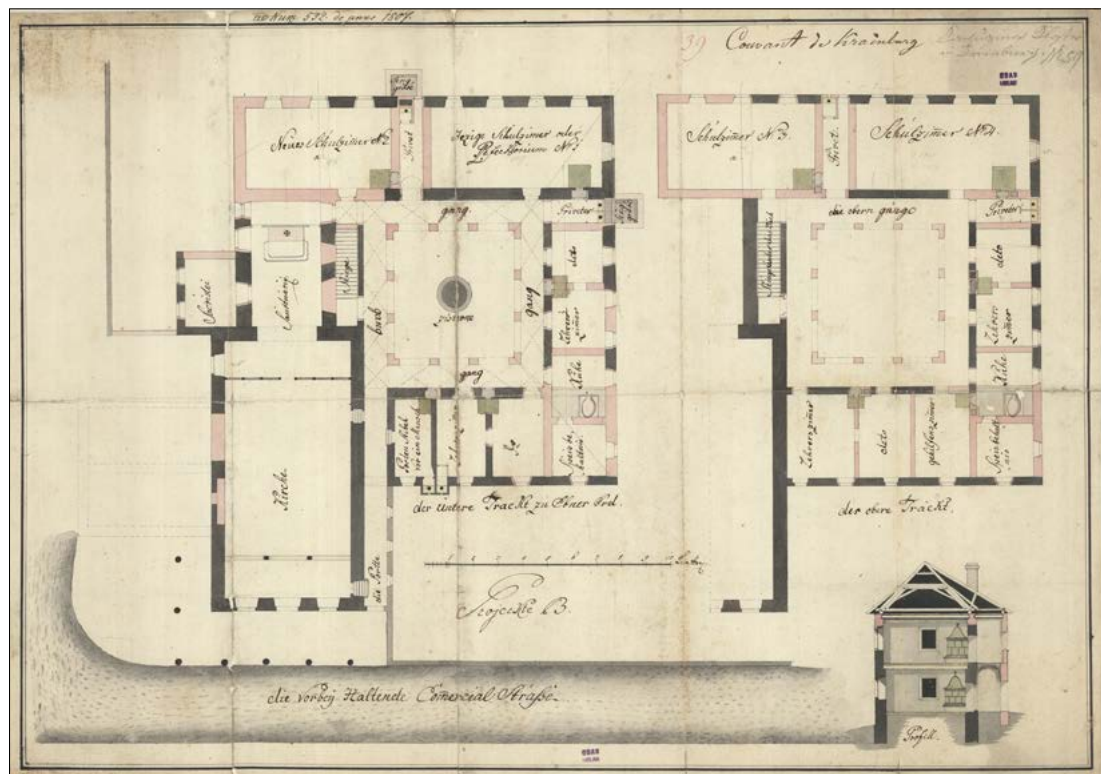
sl. 61 (zgoraj): Načrt predelave pritličja in nadstropja nekdanjega kranjskega kapucinskega samostana v vojaško kasarno (SI AS 1068, Zbirka načrtov, t. e. 300, 6/19, foto: Tanja Martelanc).
