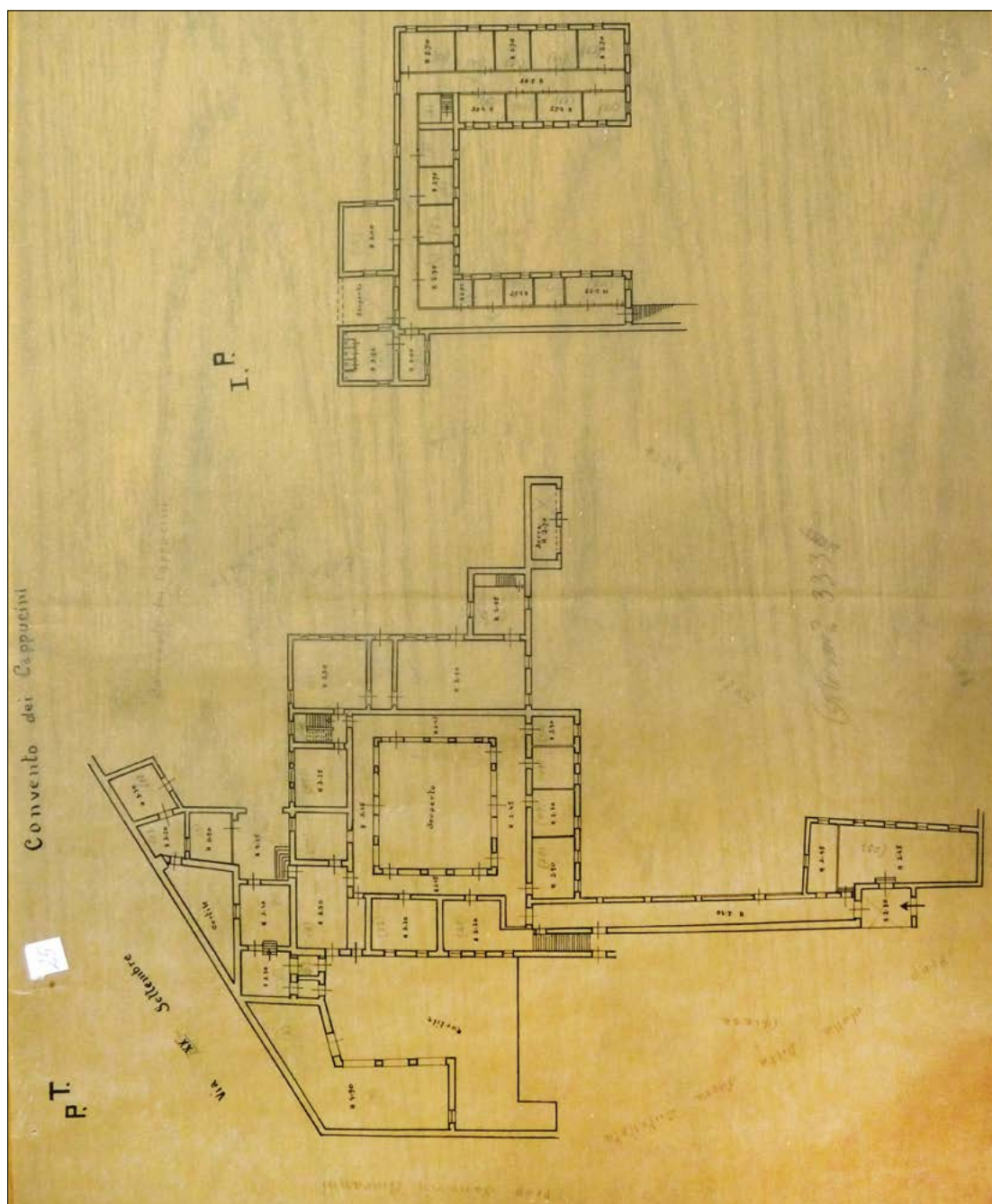
sl. 11: Pritličje in nadstropje nekdanjega koprskega kapucinskega samostana, 1852-1972 (SI_PAK/0340, Zbirka gradbenih načrtov, l. 25 (Convento dei Cappuccini), foto: Tanja Martelanc).
