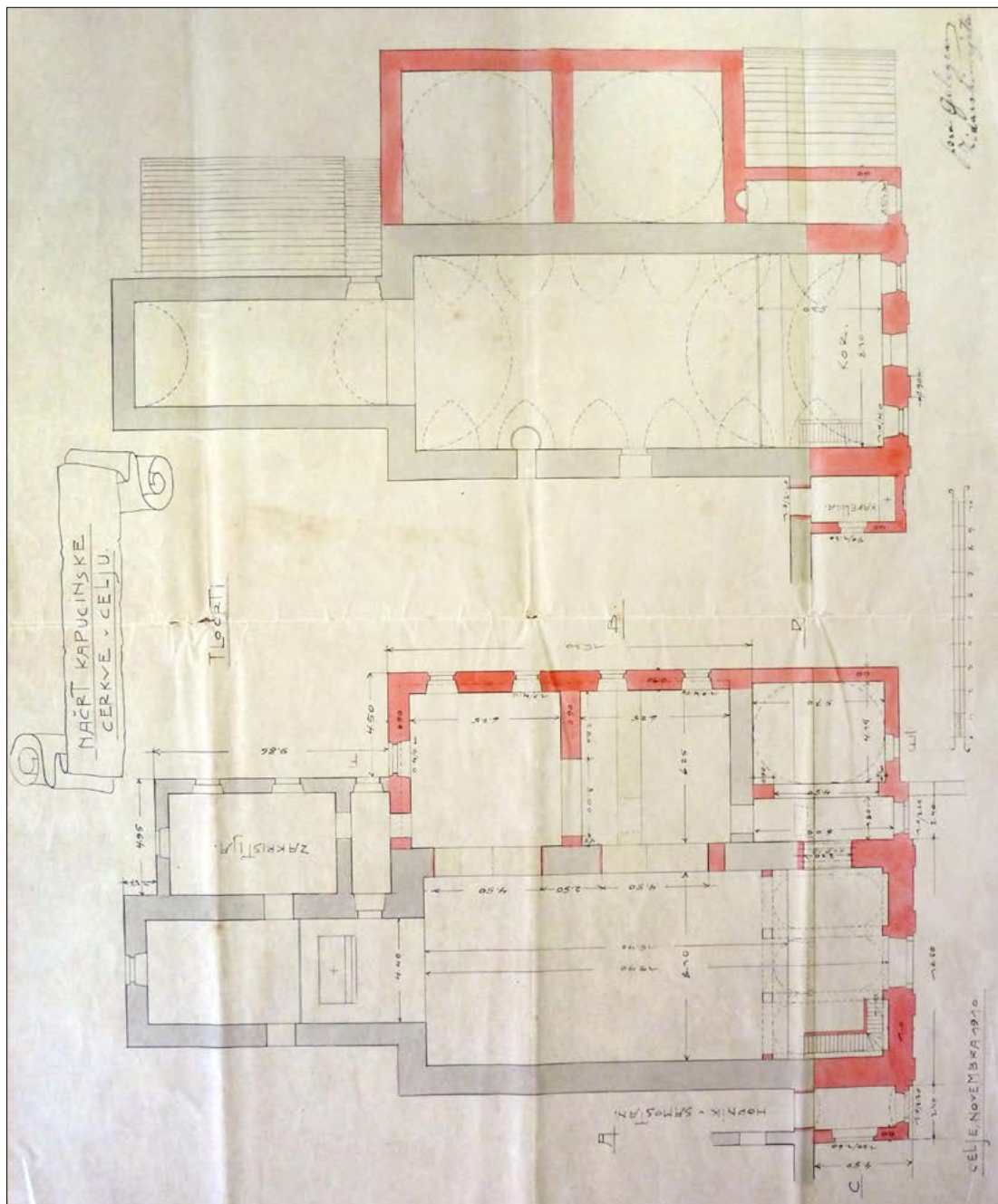
sl. 16: Načrt prenove celjske kapucinske cerkve, avtor Ferdinand Gologranc, 1910 (SI_ZAC/0024/002/022/001/00058, a. š. 111, foto: Tanja Martelanc).
