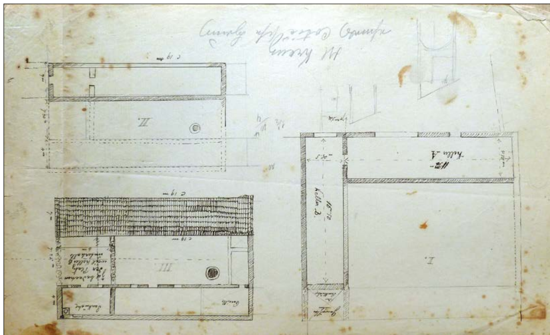
sl. 31: (zgoraj) Načrt ureditve Cotičeve hiše v gospodarska poslopja, po letu 1887 (SI ASKP, Zbirka načrtov, Svetokriški kapucinski samostan, foto: Tanja Martelanc).
