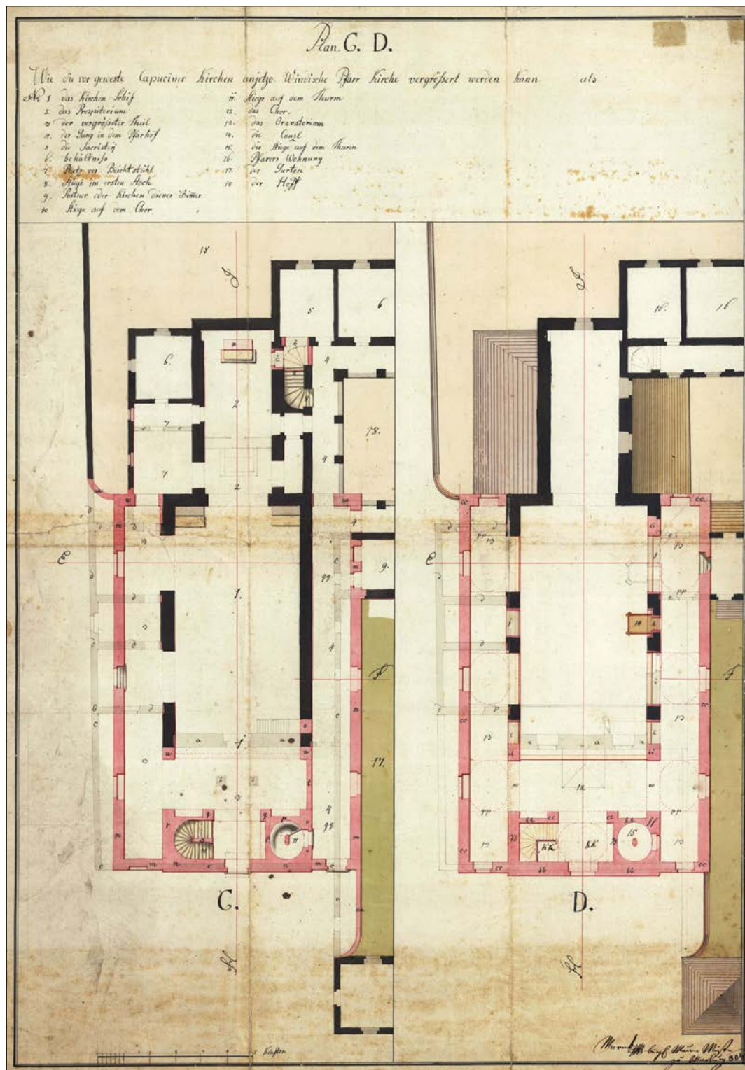
sl. 23: Načrt predvidene povečave nekdanje kapucinske cerkve v Mariboru, avtor Mihael Janez Marek, 1804 (SI_PAM/1806/001/00079).
