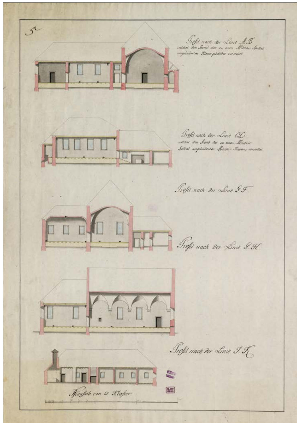
sl. 65: Prerezi predelave nekdanjega novomeškega kapucinskega samostana v bolnišnico, 1791 (SI AS 1068, Zbirka načrtov, t. e. 300, 6/203, foto: Tanja Martelanc).
