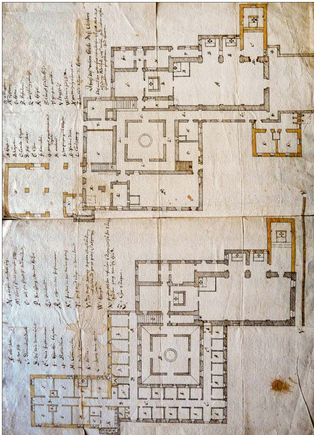
sl. 63: Načrt predelave pritličja in nadstropja novomeškega kapucinskega samostana, 1712-1713 (SI ASKP, Zbirka načrtov, Nekdanji kapucinski samostan v Novem mestu, foto: Tanja Martelanc).
