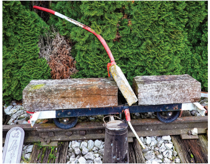
Progovni voziček modran ali madron 3 za prevoz materiala po eni tirnici.
