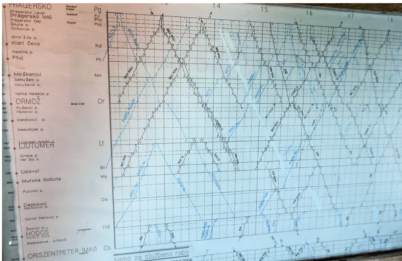
Grafikon - s črtami prikazan vozni red vlakov (navpično je razvidno ime postaje, vodoravno pa ure).
